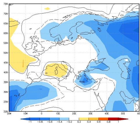
(b) La Niña, Ctrl
