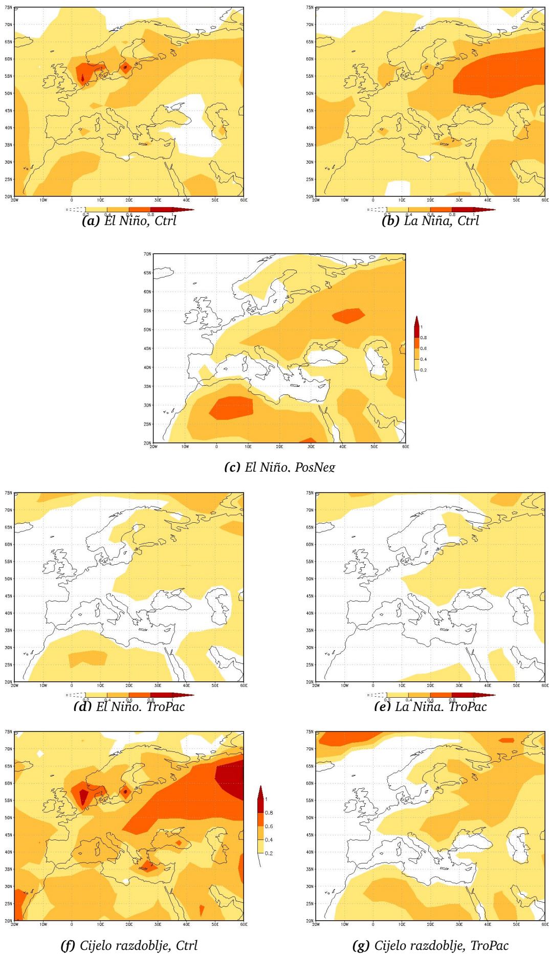
Slika 3.9: Standardna devijacija prizemne temperature za sezonu JFM
