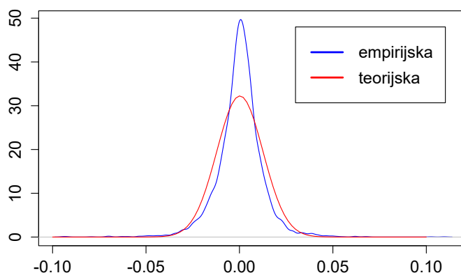
Slika 1.10: Usporedba empirijske gustoće razdiobe log-povrata i teorijske gustoće normalne razdiobe sa istom aritmetičkom sredinom i varijancom
