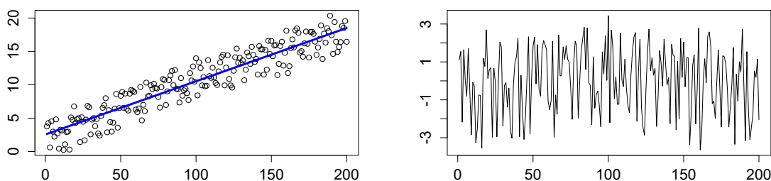
(a) Podaci i regresijska funkcija
