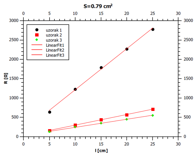
Slika 7.2: R-l graf.
