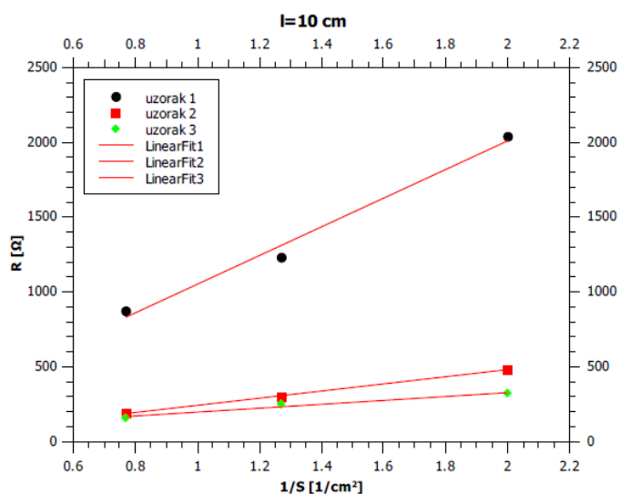
Slika 7.3: R-(1/S) graf.
