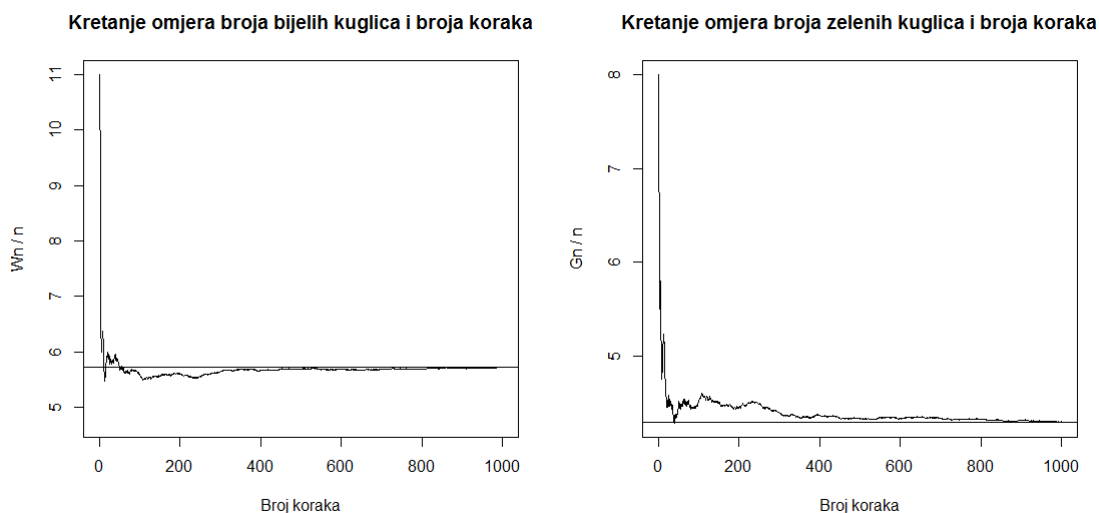
Slika 6.1: Ilustracija slabog zakona velikih brojeva za urne. Simulirano je 1000 koraka. Lijeva slika pokazuje kako se omjer \frac{W_n}{n} mijenja kroz vrijeme, a desna slika pokazuje kako se omjer \frac{G_n}{n} mijenja kroz vrijeme. Horizontalne linije predstavljaju vrijednost kojoj bi dotični omjeri trebali konvergirati. Dakle, na lijevom grafu horizontalna linija ima jednadžbu y = \lambda_1 v_1 , a na desnom grafu horizontalna linija ima jednadžbu y = \lambda_1 v_2 . Za konkretan primjer uzete su vrijednosti a = 7 , b = 3 , c = 4 , d = 6 te početni uvjeti, tj. početni broj kuglica u urni W_0 = 7 , G_0 = 2 . Valja napomenuti da početni broj bijelih i zelenih kuglica u urni ni na koji način ne utječe na asimptotski rezultat.
