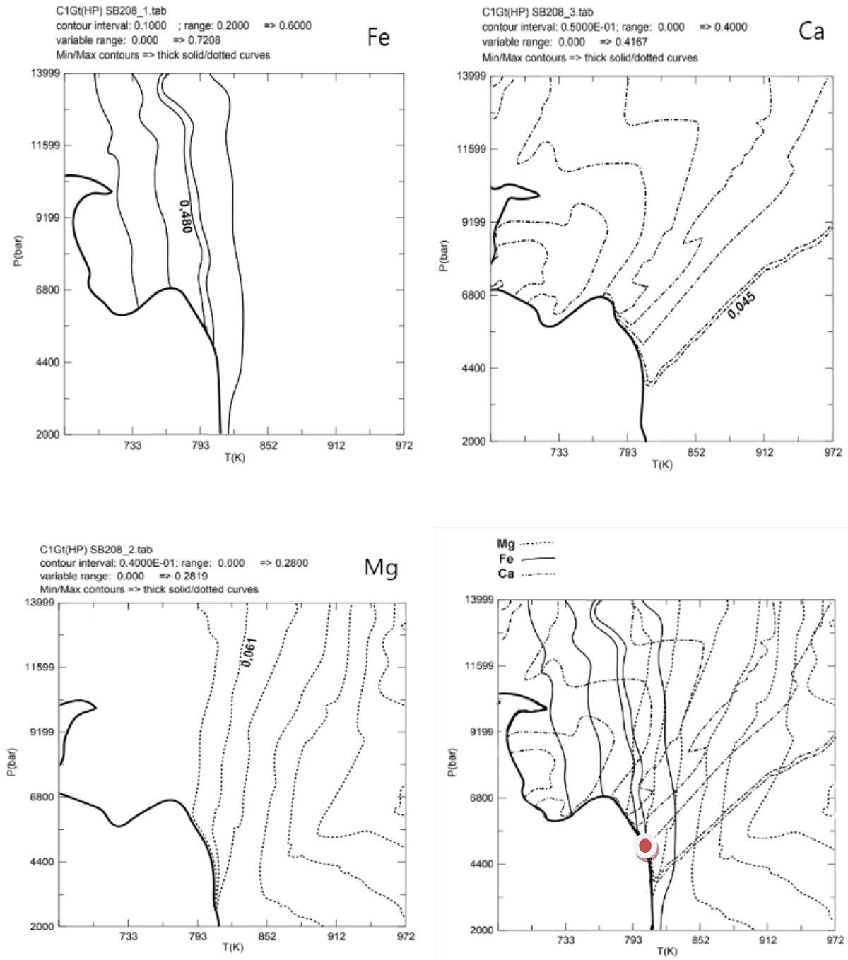
Slika 21. Izoplete Mg, Fe i Ca za granatnu analizu an2. Posljednji dijagram predstavljen s podebljanim točkom iz koje je očitana termalno-tlačna vrijednost. Izrada prema programu Perplex. Područja u donjim lijevim kvadrantima ispod podebljanih izopleta su područja gdje nema pojavnosti granata.
