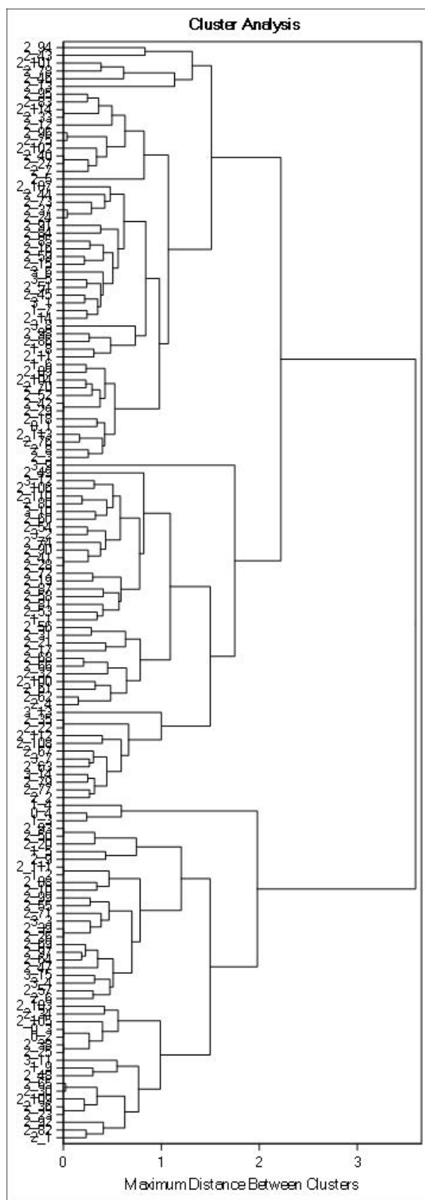
Slika 2.9: Dendrogram klsterske analize za Manhattan mjeru udaljenosti i metodu maksimuma
