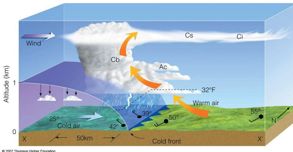
Slika 3: Nastajanje konvektivnog oblaka na hladnoj fronti (izvor: Internet)
