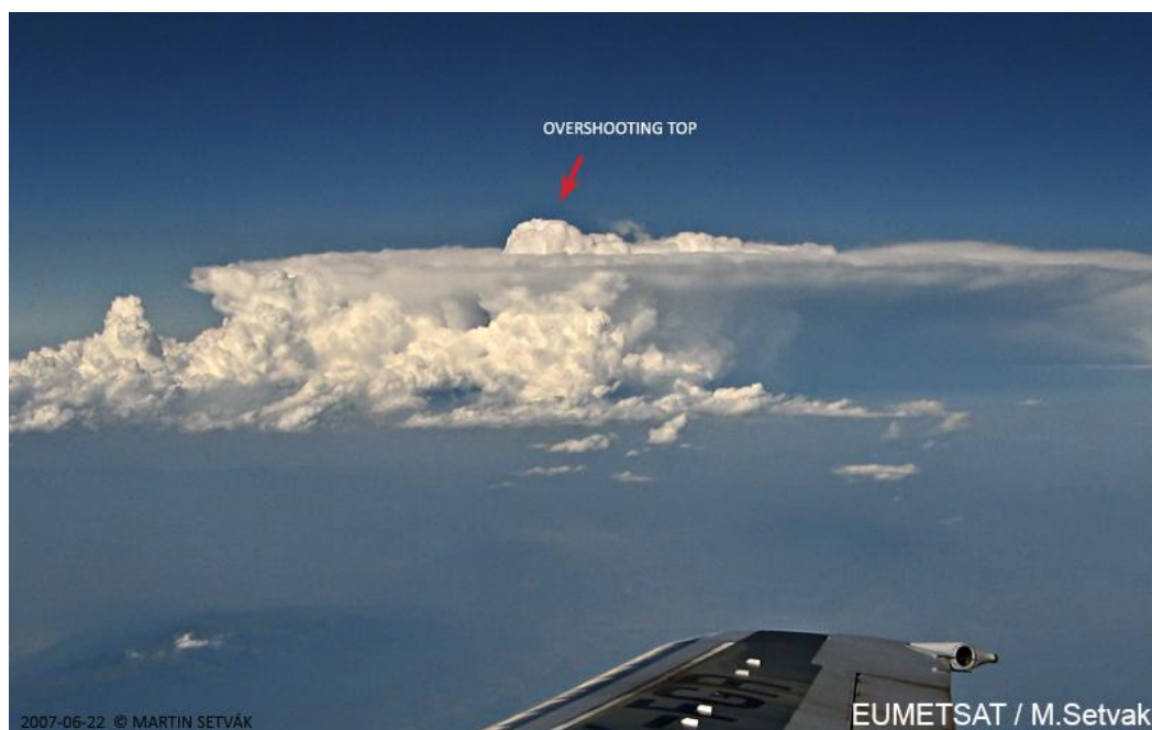
Slika 4: Primjer premašujućeg vrha (OT), fotografirano iz zrakoplova (izvor: www.convectivestorm.blogspot.hr )
