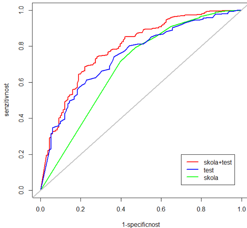
Slika 4.18: ROC krivulja
