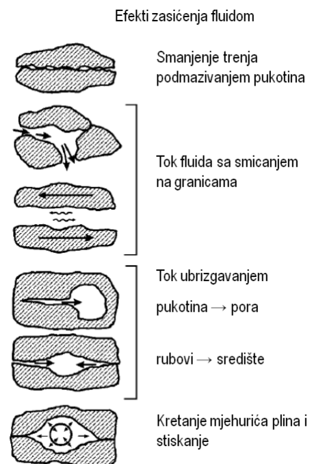
Slika 2.3 Shematski prikaz mehanizama atenuacije koji su posljedica postojanja fluida u pukotinama i porama (preuzeto i prilagođeno iz Barton, 2007).
