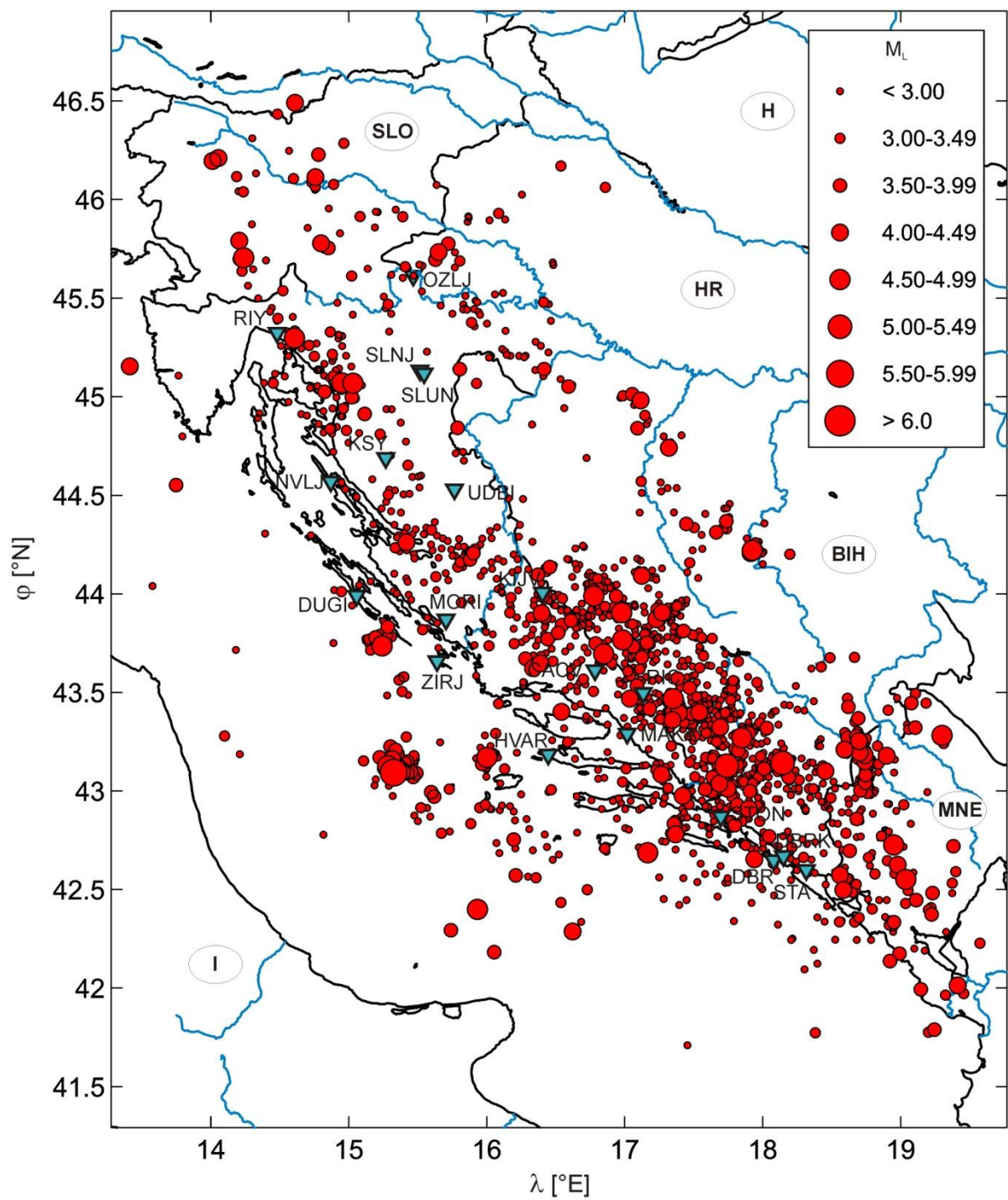
Slika 3.1 Karta epicentara korištenih potresa (crveni kružići) i seizmoloških postaja (plavi trokutići) u analizi atenuacije koda valova.
