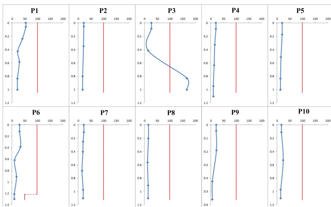
Slika 11. Raspodjela koncentracije olova (mgkg -1 ) po dubinama (m) profila P1-10.
