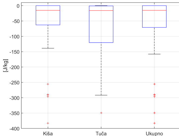
Slika 3.2: Vrijednosti SBCIN-a.
