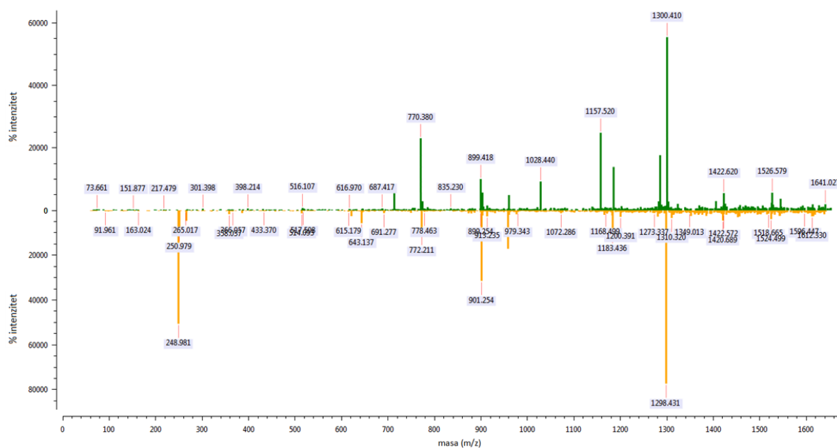
Slika 8. Prikaz MS/MS ( m/z ) spektra u pozitivnom (zeleno) i negativnom (narančasto) obliku iona za 1670.7778 peptidni fragment (proteinska mrlja 1 - protein sličan proteinu ASR3, XP_004237807, rajčica).
