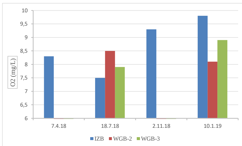
Slika 31. Koncentracija otopljenog kisika u vodi prokapnici (WGB-2 i WGB-3) i na izvoru Baračevac (IZB) iskazana u miligramima po litri
