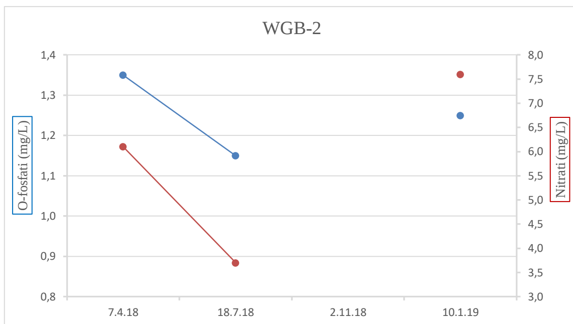
Slika 22. Koncentracija ortofosfata ( \text{PO}_4^{3-} ) i nitrata ( \text{NO}_3^- ), izražena u miligramima po litri, mjerena u vodi prokapnici (WGB-2), u razdoblju od travnja do siječnja.
