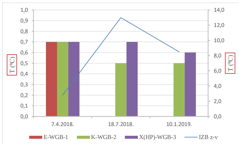
Slika 19. Temperaturna razlika između temperature zraka (E,K,X) i temperature vode prokavnice (WGB-1;2;3) te temperaturna razlika između temperature zraka i vode na izvoru Baraćevac (IZB z-v), izražena u °C
