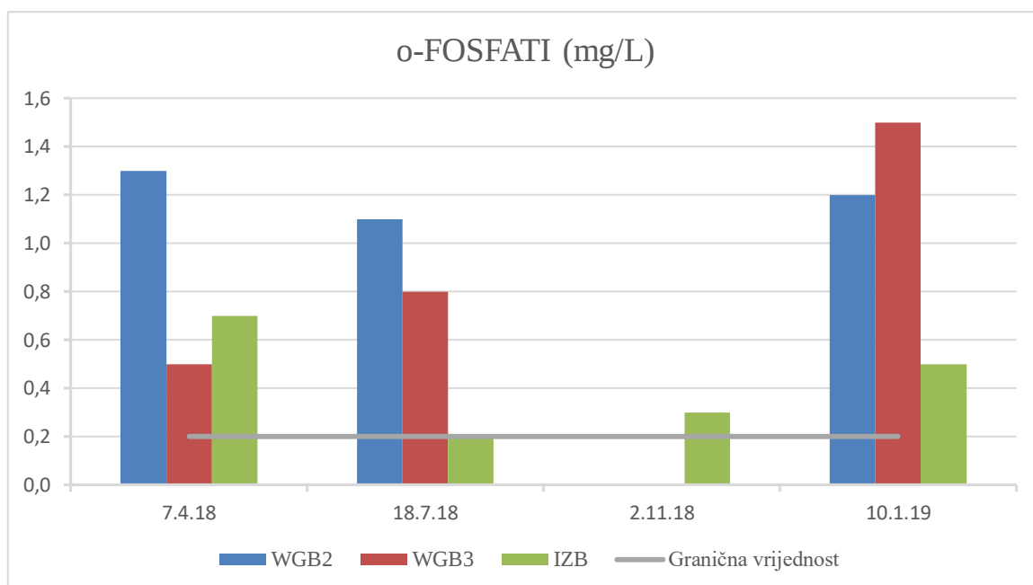
Slika 25. Koncentracija ortofosfata ( \text{PO}_4^{3-} (mg/L)) bilježena kroz vremensko razdoblje (travanj-siječanj) na svim mjeranim postajama (WGB-2, WGB-3, IZB). Linijski je pridodana granična vrijednost (prema Uredbi o izmjenama i dopunama Uredbe o standardu kakvoće voda (NN 80/2018))
