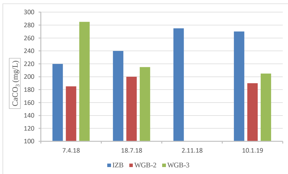
Slika 30. Vrijednosti alkaliniteta vode prokapnice (WGB-2 i WGB-3) i izvora Baračevac (IZB), iskazana u miligramima po litri
