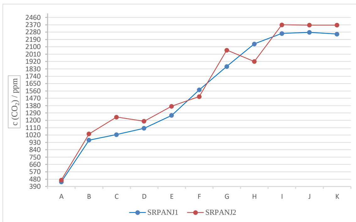
Slika 13. Raspodjela koncentracije \text{CO}_2 u zraku od točke ulaska (A) do kraja turističkog dijela špilje (K). Mjerenje je obavljeno u srpnju i izraženo u ppm.
