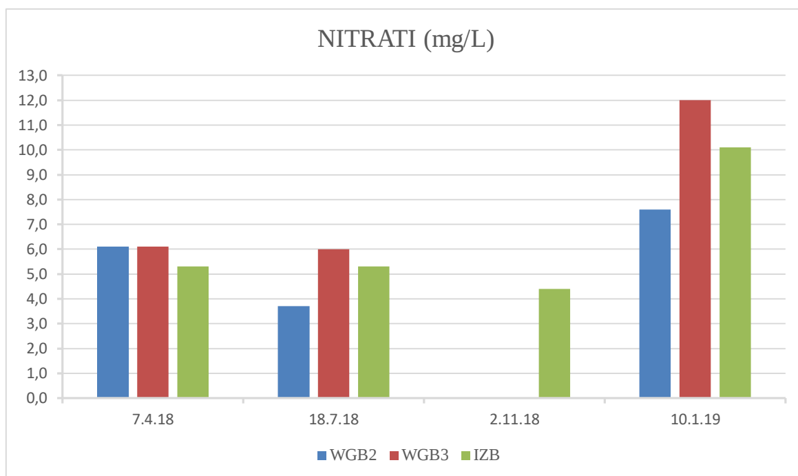
Slika 24. Koncentracija nitrata ( \text{NO}_3^- (mg/L)) kroz vremensko razdoblje (travanj-siječanj) na svim mjeranim postajama (WGB-2, WGB-3, IZB)
