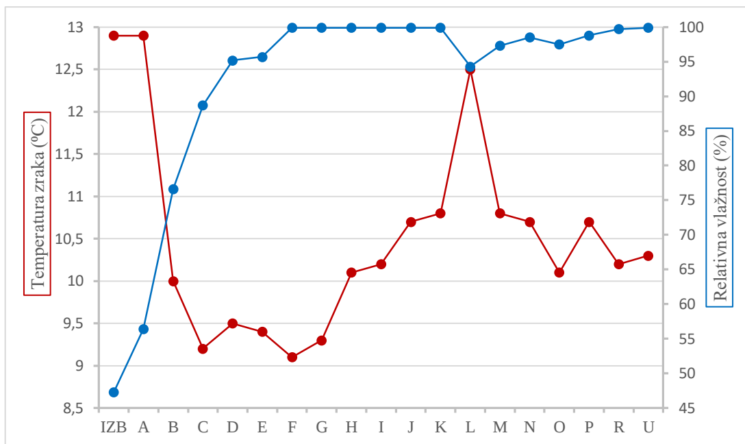
Slika 14. Odnos temperature (°C) i relativne vlažnosti zraka (%) mjerena u travnju na 19 točaka od kojih su 2 izvan (IZB, A), a ostale unutar špilje (B-U)
