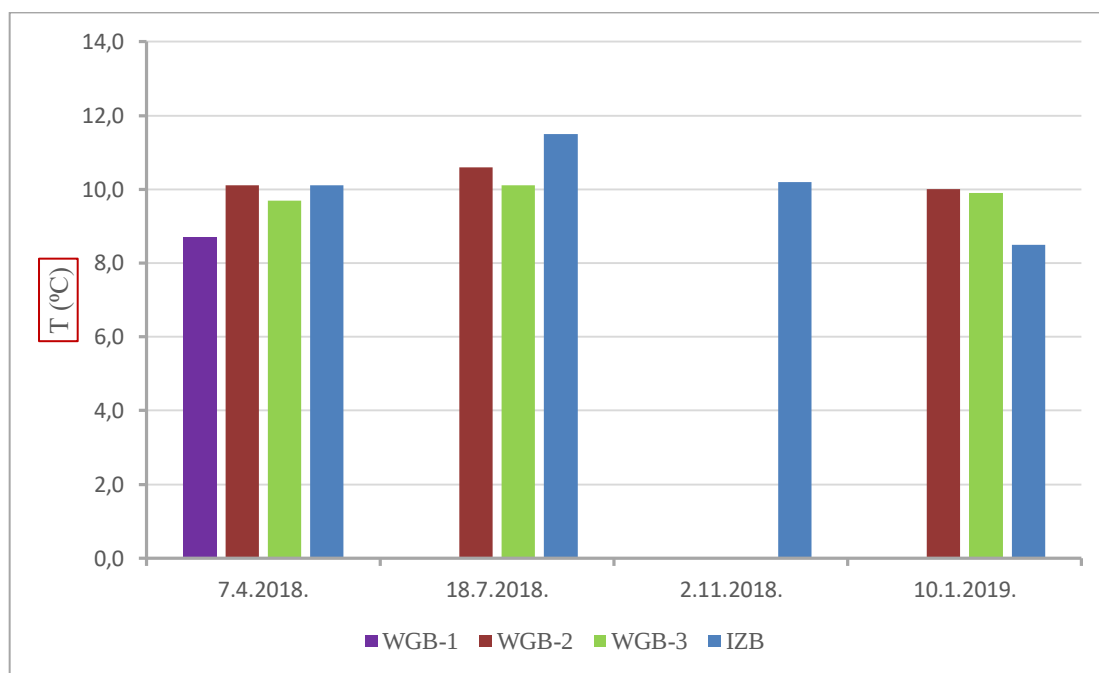
Slika 27. Odnos temperatura vode prokapsnice (WGB-1;2;3) i izvorišne vode (IZB), u mjerenim mjesecima, prikazan u °C
