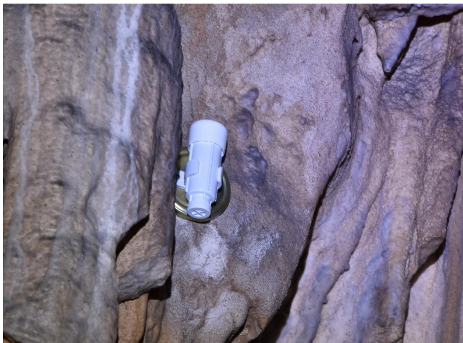
Slika 7. Memorijski termohigrograf postavljen na zid špilje
