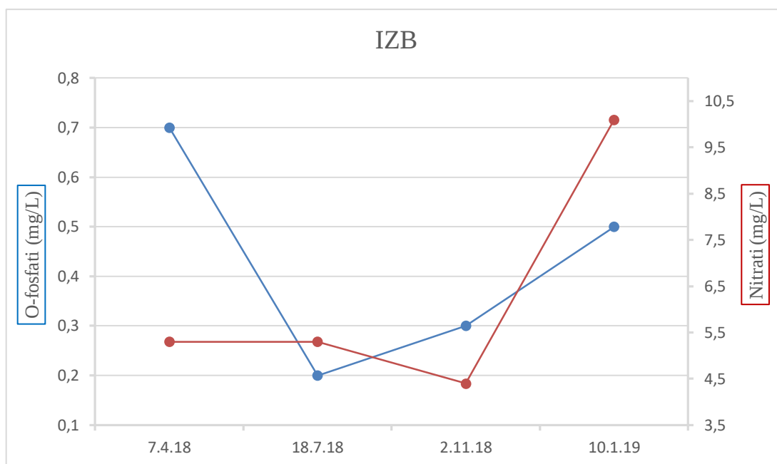
Slika 21. Koncentracija ortofosfata ( \text{PO}_4^{3-} ) i nitrata ( \text{NO}_3^- ) izražena u miligramima po litri, mjerena u izvorskoj vodi Baračevac (IZB), u razdoblju od travnja do siječnja.
