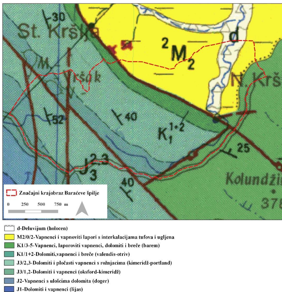
Slika 3. Geološka karta istraživnog područja Baračevih špilja (napravljena prema Polšak i dr., 1976, OGK; List Bihać, izvorno mjerilo 1:100 000)
