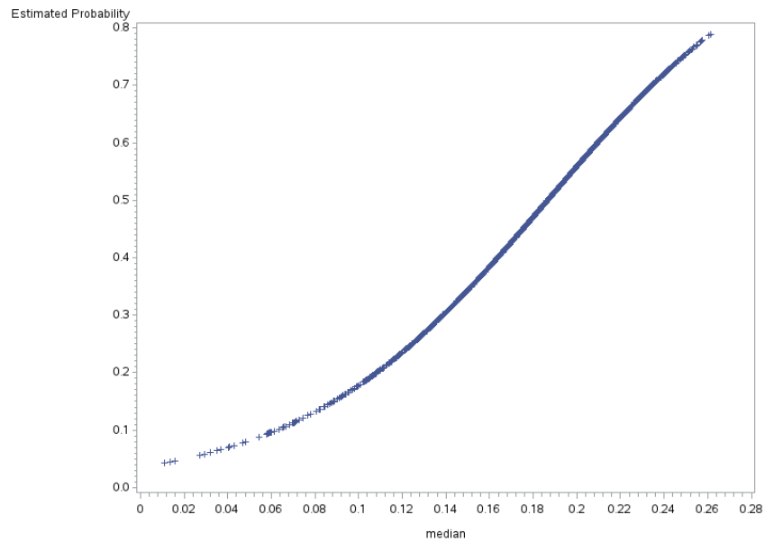
Slika 3.20: Vjerojatnost prepoznavanja ženskog glasa za varijablu median
