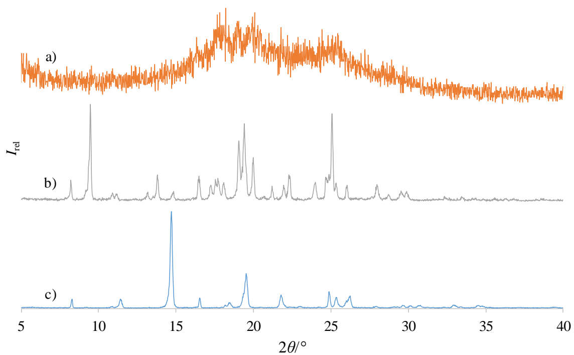
Slika 54. Usporedba difraktogramâ praškastih uzoraka a) azo mreže 5, b) triamino spoja 2, c) 4,4'-dinitrobenzila
