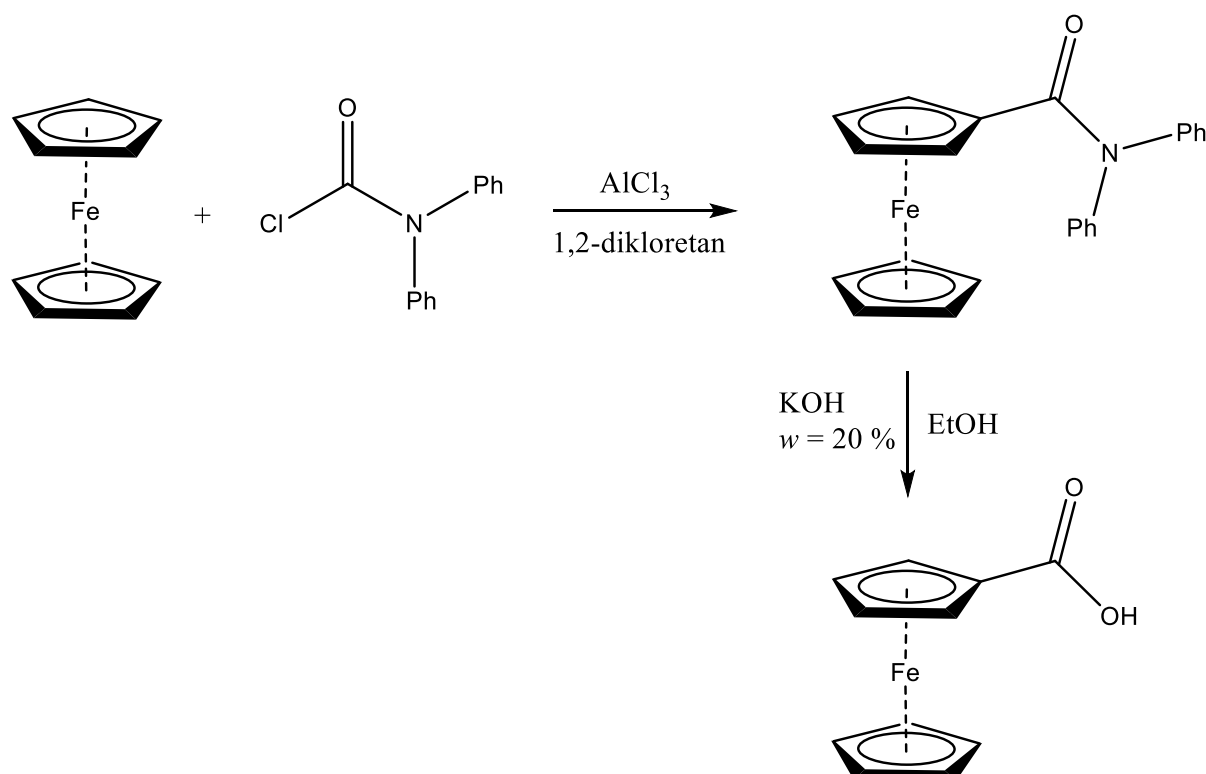
Slika 28. Shema sinteze ferocenkarkoksilne kiseline Friedel-Craftsovim aciliranjem 6
