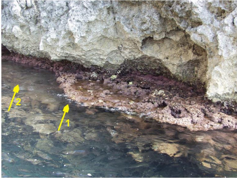
Slika 6: Prikaz morfologije alnog vijenca (trotoara) na otoku Biševu. Strelicama su označene dvije razine razvoja vijenaca: 1) gornja, 2) donja (preuzeto iz Faivre et al., 2013).
