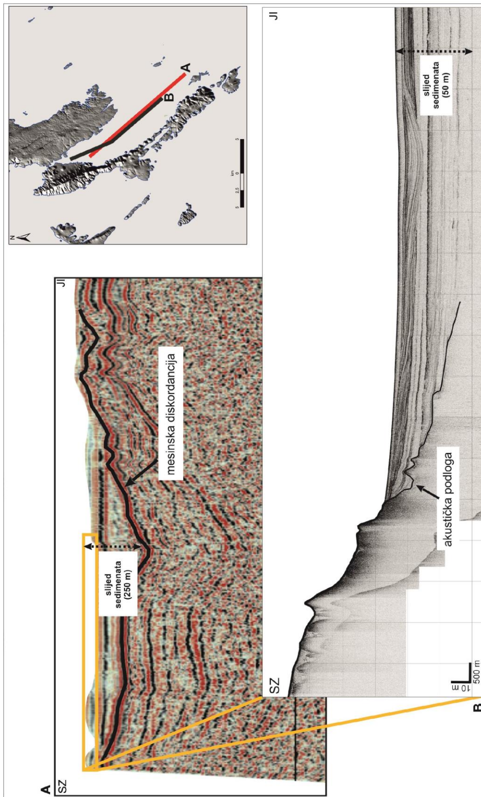
Slika 114: Profil duboke seizmike (Durn, 2016) (A) i seizmički profil visoke rezolucije (B) s prostora Lošinjškoga kanala. A) Tektonski uvjetovana depresija u kršu s označenom mesinskom diskordancijom, te sedimentnim slijedom debljine oko 250 m. B) Prikaz najgornjih 50 m slijeda sedimentata visoke rezolucije. Akustička podloga na profilu odgovara okršnim karbonatnim stijenama prisutnim i na okolnim otocima.
