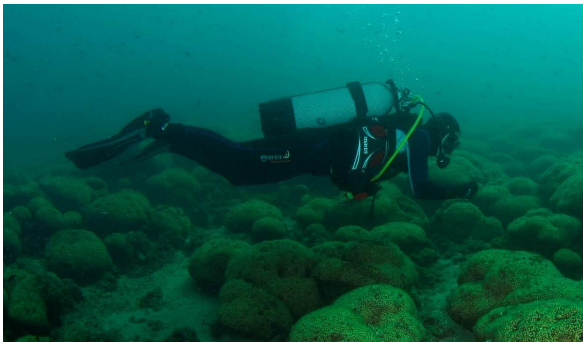
Slika 12. Istraživanje grebena koralja Cladocora caespitosa u Velikom jezeru (NP Mljet).
