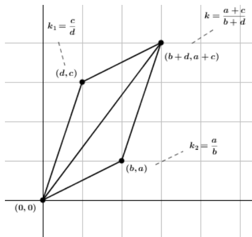
Slika 3.1: Grafički prikaz svojstva (1)
