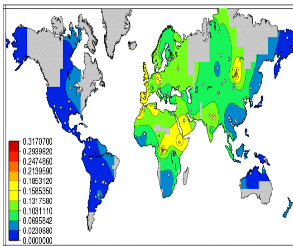
Slika 12. Raspodjela alela HLA DRB1*07:01 u svijetu (preuzeto iz [16])
