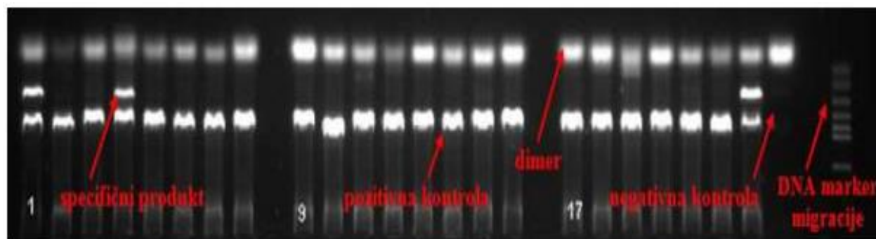
Slika 20. Fotografija agaroznog gela s produktima PCR
