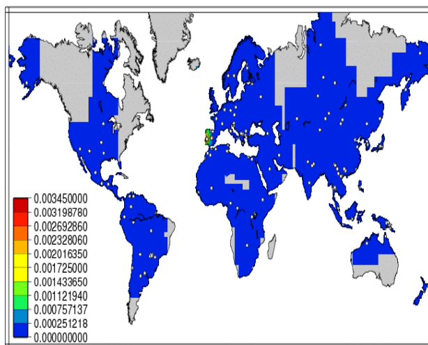
Slika 12. Raspodjela alela HLA DRB1*07:01 u svijetu (preuzeto iz [16])
