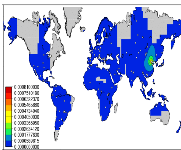
Slika 13. Raspodjela alela HLA DRB1*07:03 u svijetu (preuzeto iz [16])
