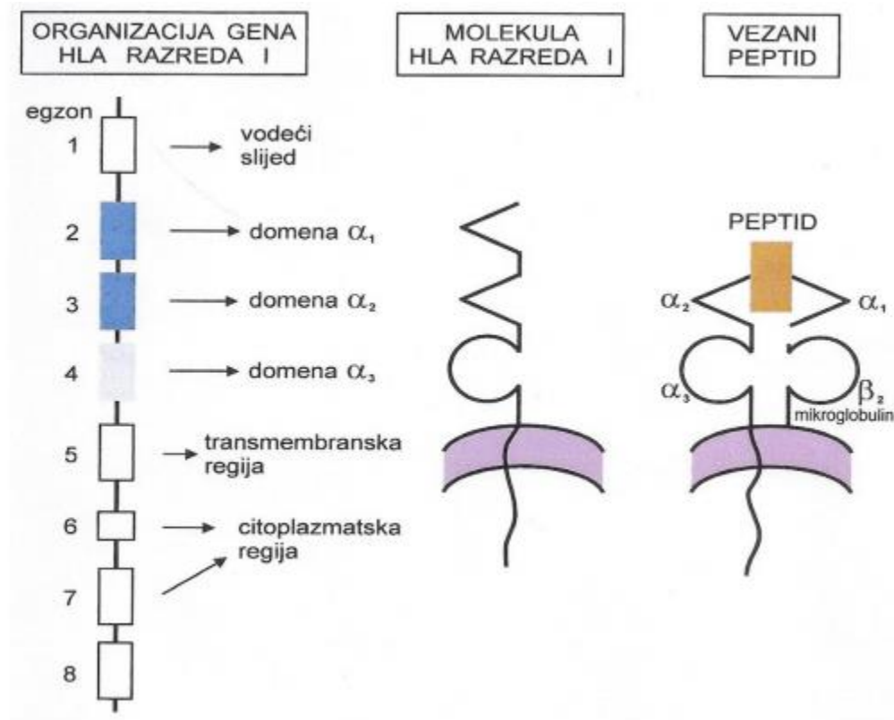
Slika 4. Shematski prikaz organizacije gena i molekule HLA razreda I (preuzeto iz [2])
