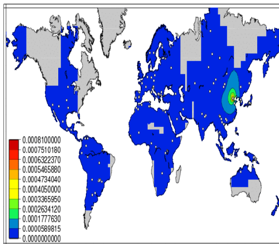
Slika 13. Raspodjela alela HLA DRB1*07:03 u svijetu (preuzeto iz [16])
