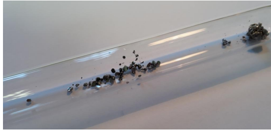
Slika 5.1.3: Fotografija ampule s Cd 3 As 2 nakon završene sinteze. Izrasli kristali su izolirani i koncentrirani su oko sredine ampule, gdje je u trenutku početka sublimacije početnog materijala temperatura bila najniža.
