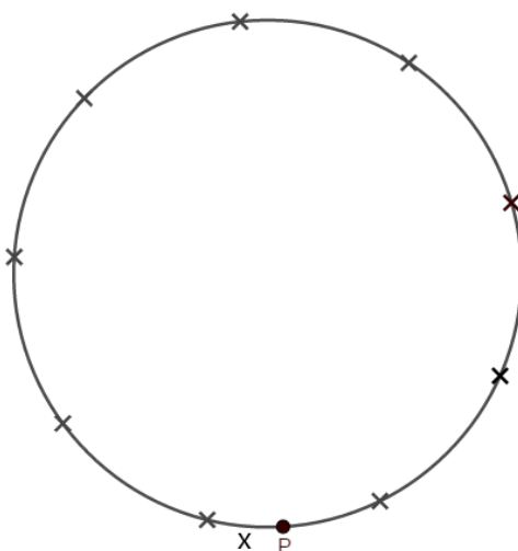
Slika 2.3: Kružni sustav od N = 9 zvijezda
