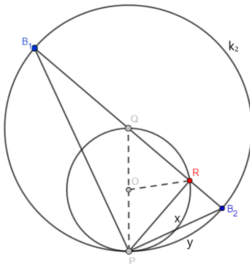
Slika 2.6: Zamjena jedne zvijezde dvjema zvijezdama
