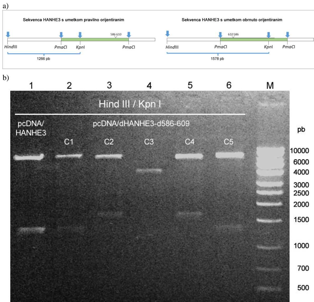
Slika 15. Ispitivanje orijentacije umetka unutar mutiranog plazmida pcDNA/dHA-NHE3 restrikcijjskim endonukleazama. a) Shematski su prikazane sekvenca HA-NHE3 s umetkom (označen zeleno). Na lijevoj strani sheme je sekvenca HA-NHE3 s pravilno orijentiranim umetkom, dok se na desnoj strani nalazi sekvenca HA-NHE3 s obrnuto orijentiranim umetkom. Kod pravilno orijentiranog umetka nakon inkubacije HA-NHE3 s endonukleazama HindIII i KpnI nastaje fragment dug 1266 pb, dok kod obrnuto orijentiranog umetka nastaje fragment dug 1578 pb. b) Prikazana je elektroforeza mutiranih plazmida pcDNA/dHA-NHE3 izoliranih iz pet različitih kolonija (linije 2-6) i inkubiranih s endonukleazama HindIII/KpnI . U plazmidima izoliranim iz C1 (linija 2) i C5 (linija 6) kolonija nastaje DNA fragment dug ~1300 pb što sugerira da je umetak pravilno orijentiran. U ostalim kolonijama nalazi ukazuju da je umetak obrnuto orijentiran unutar mutiranog plazmida pcDNA/dHA-NHE3 . U liniji 1 je nemutirani plazmid pcDNA/HA-NHE3 inkubiran s HindIII/KpnI koji služi kao kontrola. M - označava 1 kb marker DNA.
