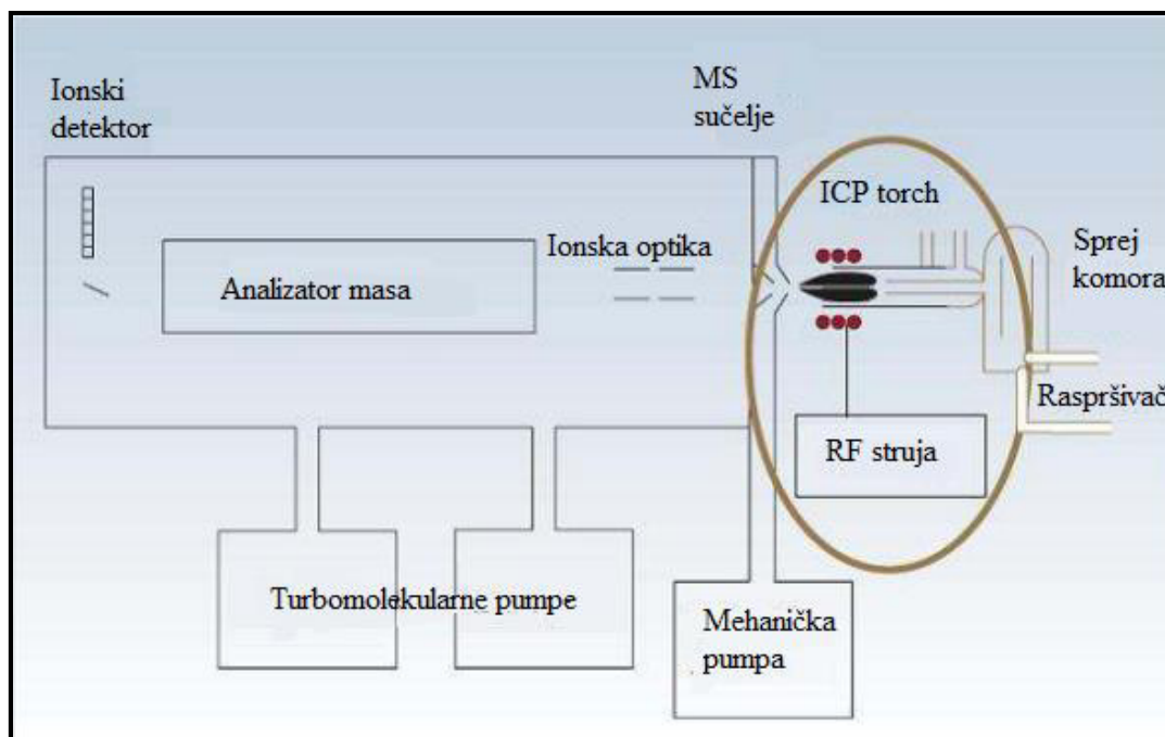
Slika 9. Shematski prikaz ICP-MS-a
