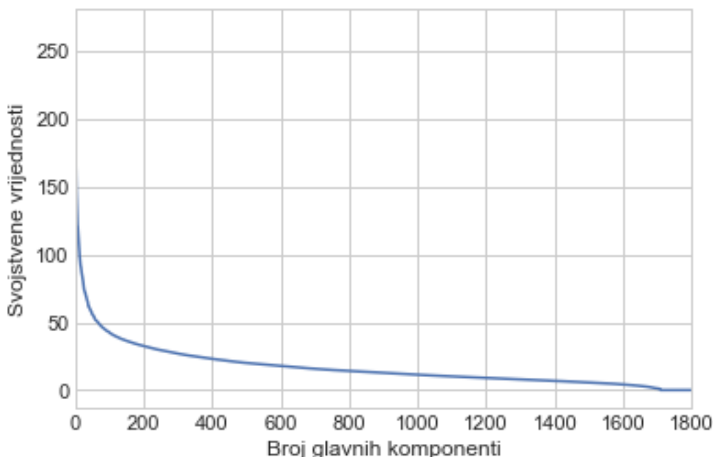
Slika 6.1: Svojtvene vrijednosti
