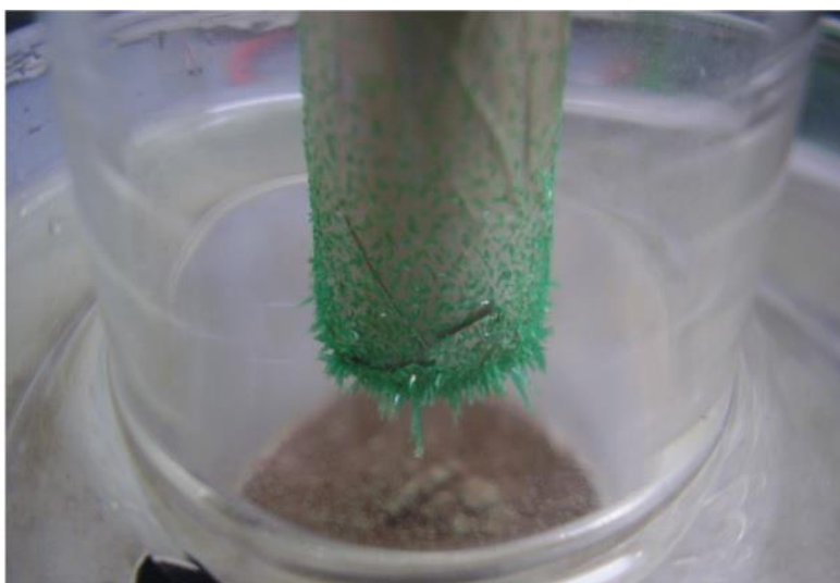
Slika 9. Odvajanje p -jodnitrobenzena sublimacijom nakon mehanokemijske sinteze 10
