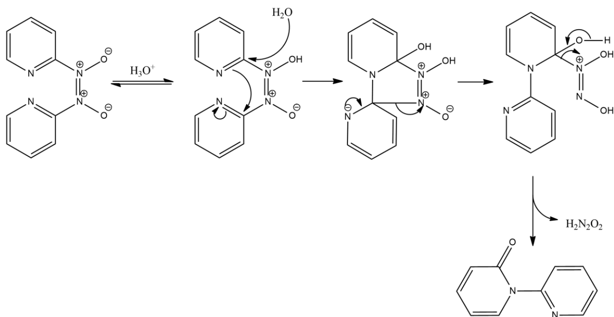
Slika 20. Mehanizam hidrolize dimera 2-nitrozopiridina
