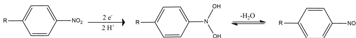
Slika 6. Redukcija aromatskog C-nitro spoja u ozračevoj TiO 2 suspenziji
