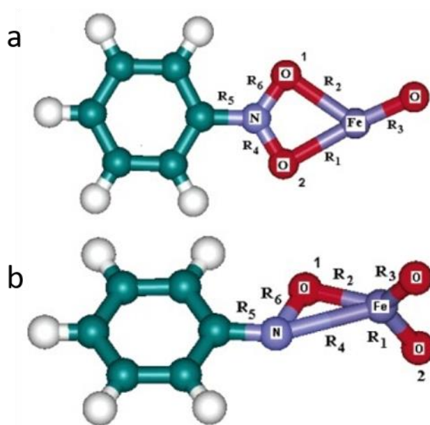
Slika 1. Međuprodukti formirani tijekom interakcije nitrobenzena i željezovog monoksida (struktura a) i nitrozobenzena i željezovog dioksida (struktura b) 4
