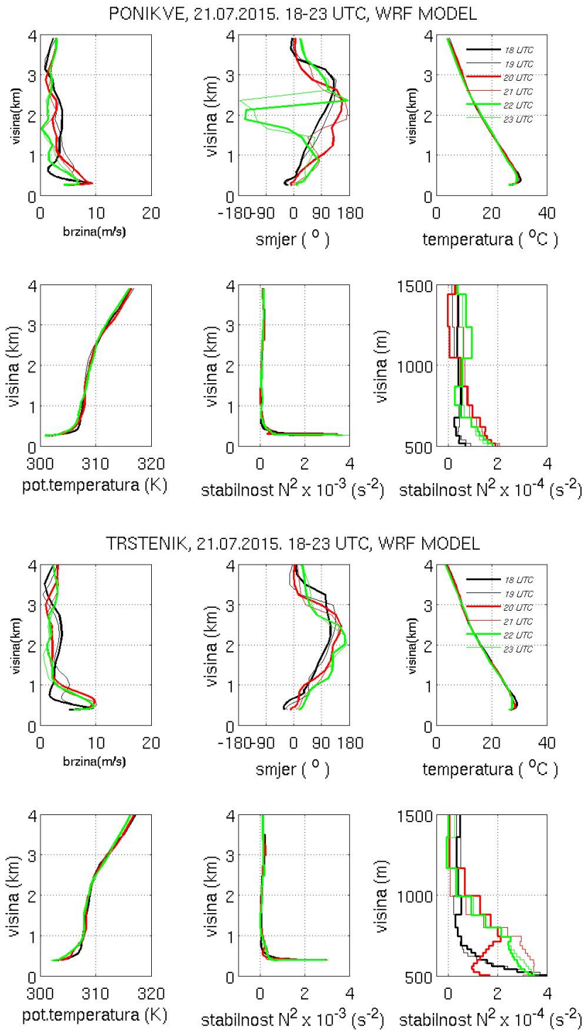
Slika 6.10: Vertikalni profili brzine vjetrova (gore lijevo), smjera vjetrova (gore sredina), temperature zraka (gore desno), potencijalne temperature (dolje lijevo), kvadrata uzgonske frekvencije (dolje sredina) i uvećani profil kvadrata uzgonske frekvencije (dolje desno) za Ponikve (slika gore) i Trstenik (slika dolje) 21.7.2015. od 18 do 23 UTC dobiveni modelom WRF.
