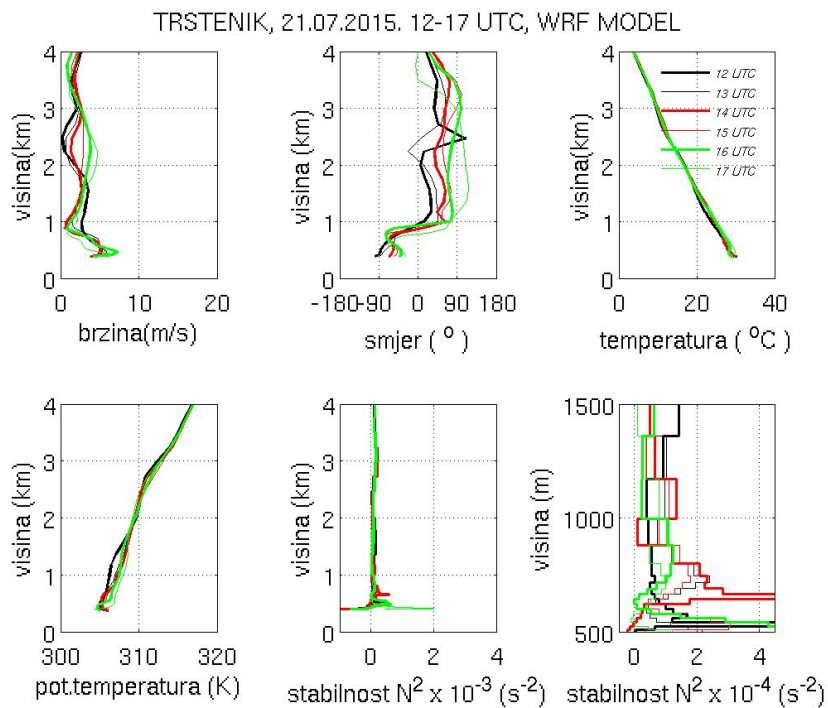
Slika 6.9: Vertikalni profili brzine vjeta (gore lijevo), smjera vjeta (gore sredina), temperature zraka (gore desno), potencijalne temperature (dolje lijevo), kvadrata uzgonske frekvencije (dolje sredina) i uvećani profil kvadrata uzgonske frekvencije (dolje desno) za Ponikve (slika gore) i Trstenik (slika dolje) 21.7.2015. od 12 do 17 UTC dobiveni modelom WRF.
