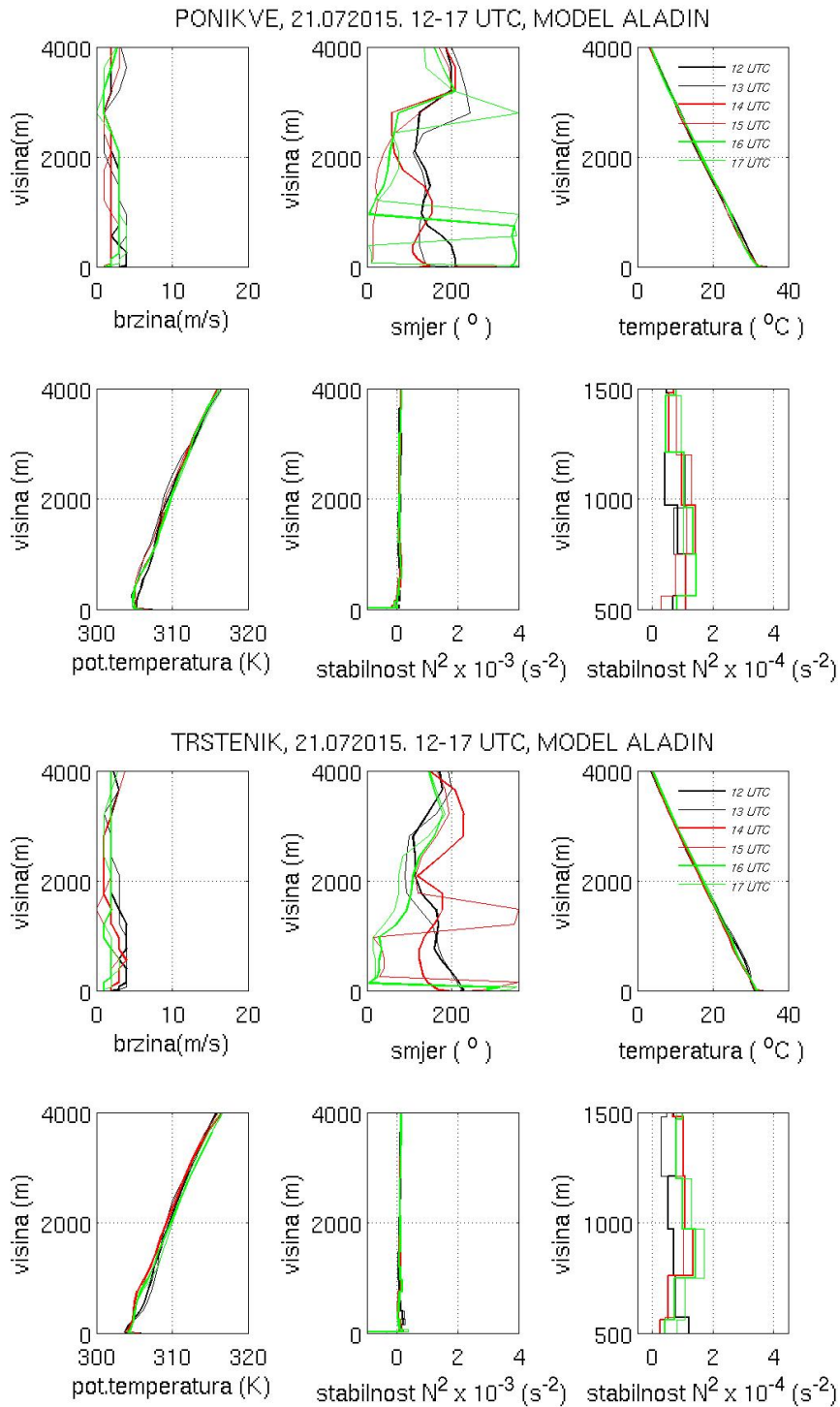
Slika 6.12: Vertikalni profili brzine vjetrova (gore lijevo), smjera vjetrova (gore sredina), temperature zraka (gore desno), potencijalne temperature (dolje lijevo), kvadrata uzgonske frekvencije (dolje sredina) i uvećani profil kvadrata uzgonske frekvencije (dolje desno) za Ponikve (slika gore) i Trstenik (slika dolje) 21.7.2015. od 12 do 17 UTC dobiveni modelom ALADIN/HR.
