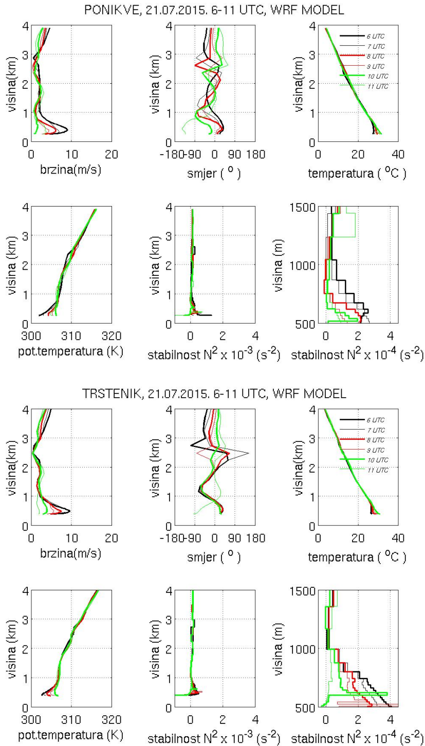
Slika 6.8: Vertikalni profili brzine vjeta (gore lijevo), smjera vjeta (gore sredina), temperature zraka (gore desno), potencijalne temperature (dolje lijevo), kvadrata uzgonske frekvencije (dolje sredina) i uvećani profil kvadrata uzgonske frekvencije (dolje desno) za Ponikve (slika gore) i Trstenik (slika dolje) 21.7.2015. od 6 do 11 UTC dobiveni modelom WRF.
