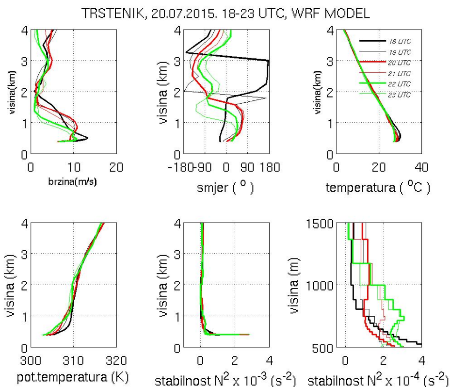
Slika 4.26: Vertikalni profili brzine vjetrova (gore lijevo), smjera vjetrova (gore sredina), temperature zraka (gore desno), potencijalne temperature (dolje lijevo), kvadrata uzgonske frekvencije (dolje sredina) i uvećani profil kvadrata uzgonske frekvencije (dolje desno) za Ponikve (slika gore) i Trstenik (slika dolje) 20.7.2015. od 18 do 23 UTC dobiveni modelom WRF.
