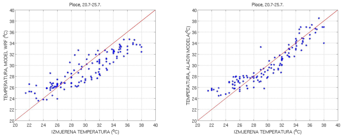
Slika 4.19: Usporedba izmjerenih temperatura zraka i simuliranih modelima WRF (lijevo) i ALADIN (desno) u razdoblju 20.–25. srpnja 2015.
