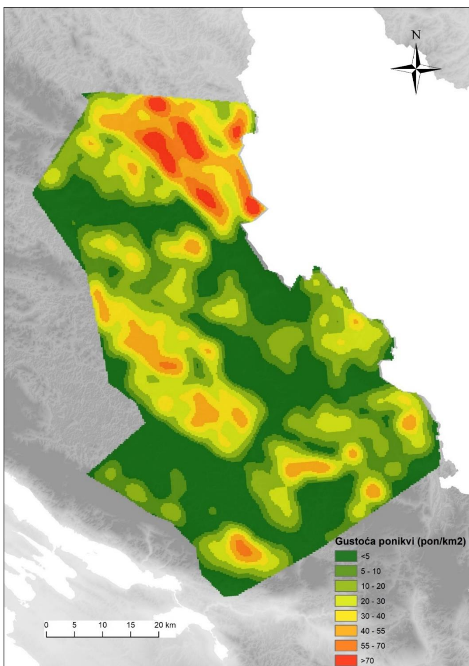
Slika 16: Gustoća ponikvi
