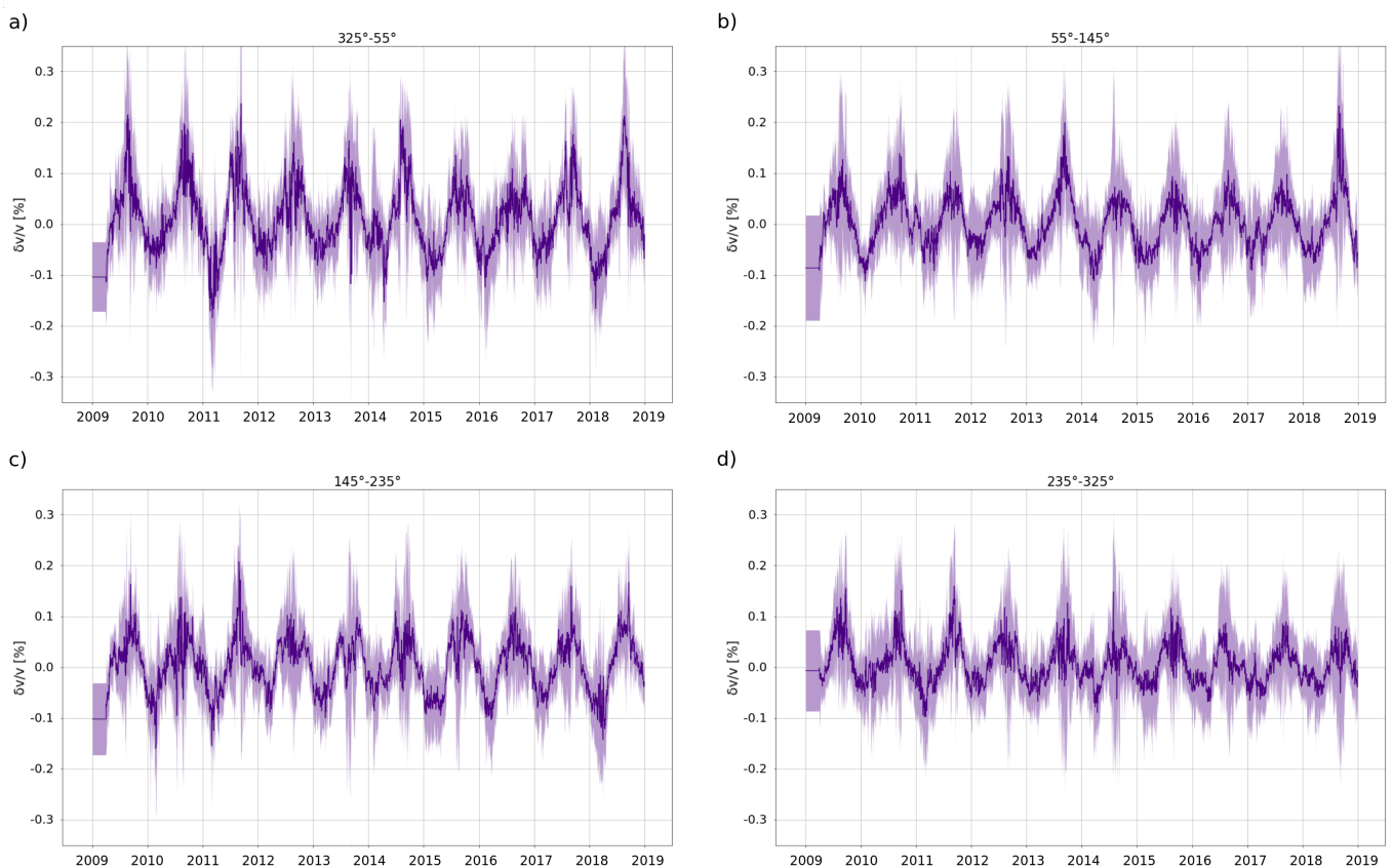
Slika 5.7: Medijalne vrijednosti \delta v/v (ljubičaste krivulje) i njihova odstupanja (svijetlo ljubičasta naznačena područja) dobivena u frekventnom rasponu 0.125–0.33 Hz za: a) prvu (azimuti 325°–55°), b) drugu (55°–145°), c) treću (145°–235°) i d) četvrtu grupu (azimuti 235°–325°) parova postaja.
