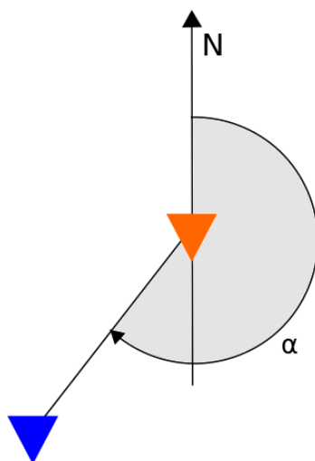
Slika 5.6: Skica načina na koji je za par postaja određen azimut smjera propagiranja signala. Kut \alpha (azimut smjera iz kojeg dolazi signal) mjeri se od sjevera (N) u smjeru kazaljke na satu kao što je naznačeno sivom bojom - za slučaj na slici azimut plave postaje u odnosu na narančastu iznosio bi oko 220^{\circ} .
