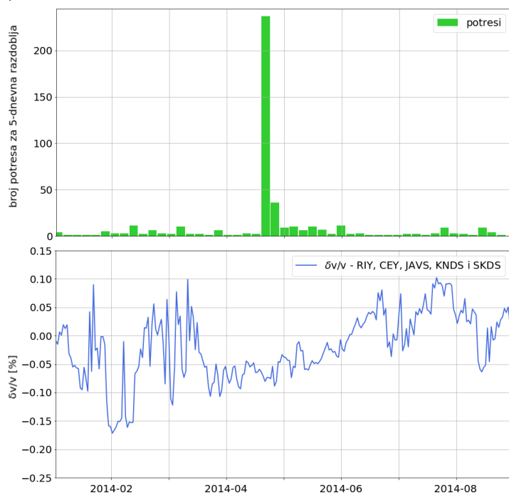
Slika C.16: Histogram broja potresa za petodnevna razdoblja i modificirani grafovi koji se odnose na: a) područje koje obuhvaća petu seriju potresa; b) čitavo analizirano područje.
