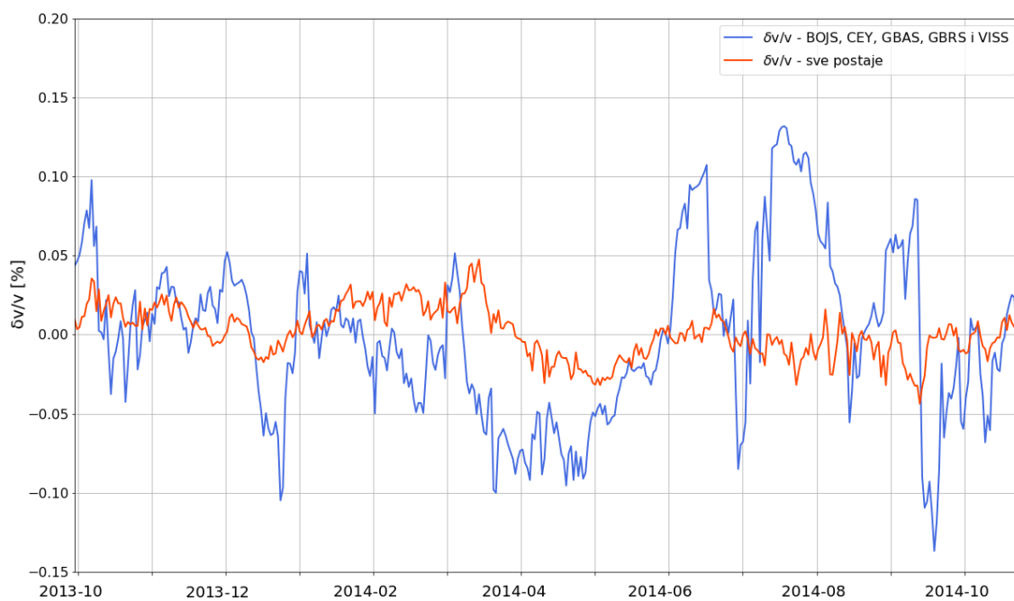
Slika C.12: Modificirane \delta v/v krivulje koje se odnose na čitavo analizirano područje i područje koje uključuje četvrtu seriju potresa.
