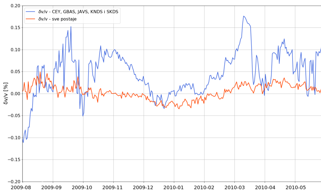
Slika C.4: Modificirane \delta v/v krivulje koje se odnose na čitavo analizirano područje i područje koje uključuje drugu seriju potresa.
