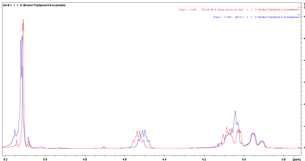
Slika 27. Preklapljeni ^1\text{H} NMR spektri propargiliranih dipeptida dobivenih metodama I (plavo) i II (crveno).
