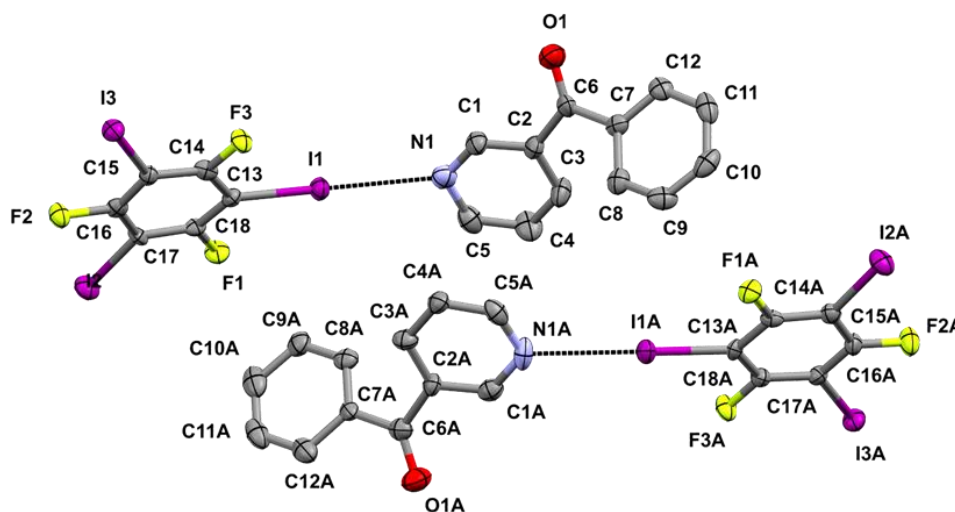
Slika 27. ORTEP prikaz strukture asimetrične jedinice (3bzy)(135titfb) s označenim atomima i halogenskom vezom. Elipsoidi svih atoma prikazani su na razini vjerojatnosti od 25 %. Vodikovi atomi nisu prikazani radi bolje preglednosti.
