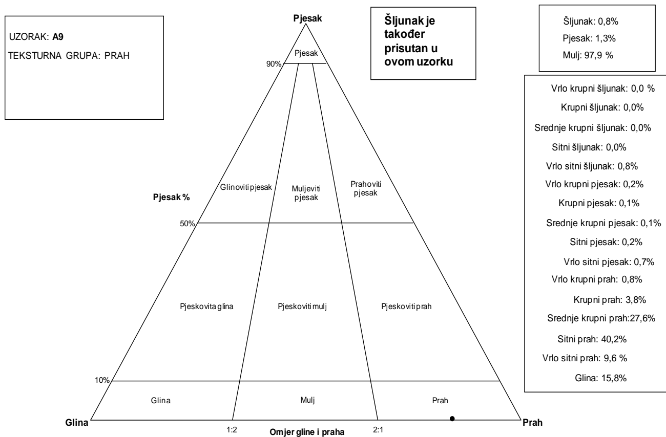
Slika 12. Trokomponentni dijagram za uzorak A-9.
