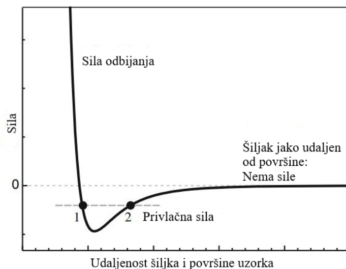
Slika 3. Djelovanje sile između šiljka i površine uzorka u ovisnosti o njihovoj međusobnoj udaljenosti opisano pomoću Lennard-Jonesovog potencijala (preuzeto iz B. Voigtländer, Scanning Probe Microscopy , Springer-Verlag, Berlin, 2015. str. 8)
