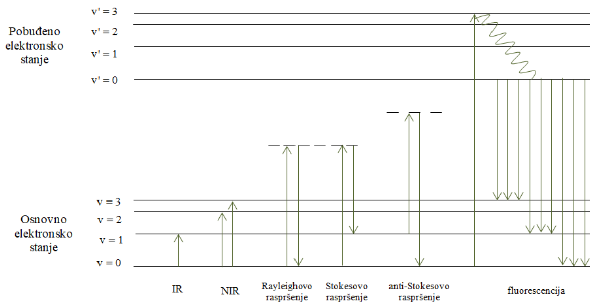
Slika 2. Shematski prikaz IR i NIR apsorpcije, Rayleighovog, Stokesovog i anti-Stokesovog raspršenja te fluorescencije
