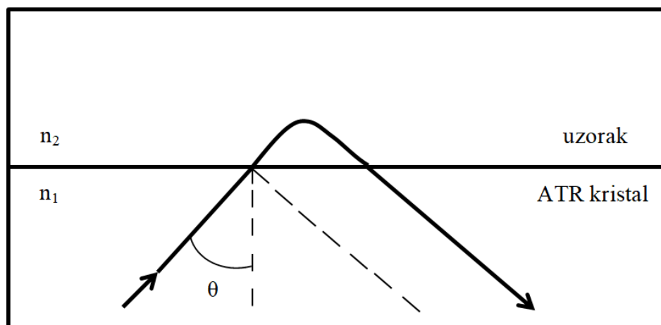
Slika 4. Shema prigušene totalne refleksije
