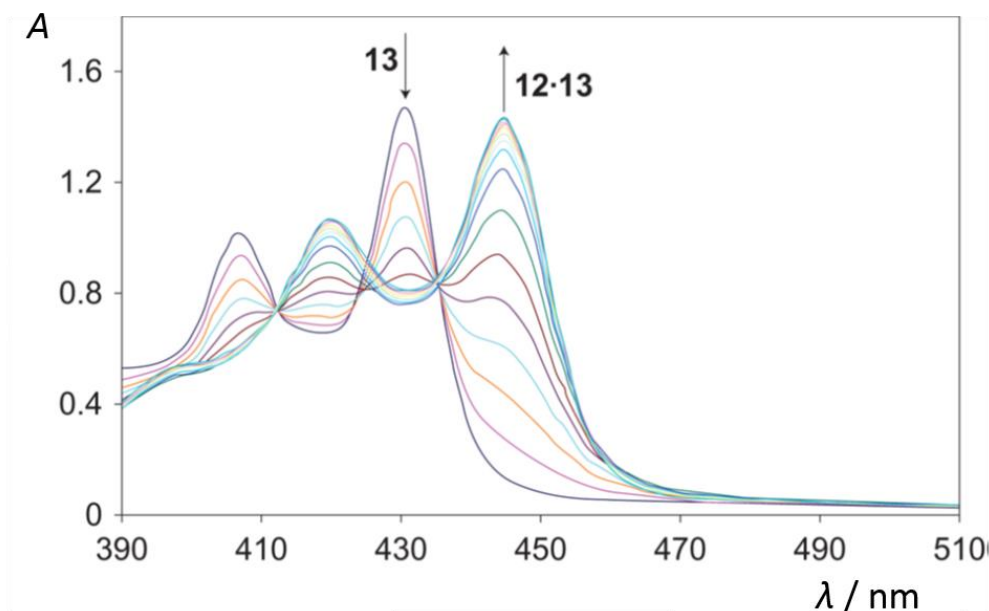
Slika 11. UV-Vis titracija AAAA(13) ( c \sim 5 \times 10^{-5} \text{ mol dm}^{-3} ) s DDDD + (12) (0-5 ekvivalenata) u CH 2 Cl 2 održavajući stalnu koncentraciju (13) pri T = 298 \text{ K} (ref. 51)
