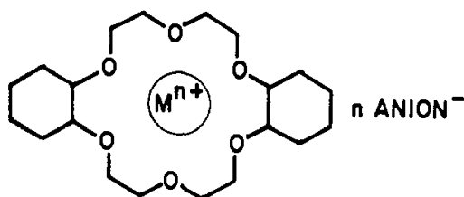
Slika 19. Shematski prikaz strukture kompleksa krunastog etera dicikloheksil-18-kruna-6 s kationom metala, \text{M}^{n+} (ref. 58)
