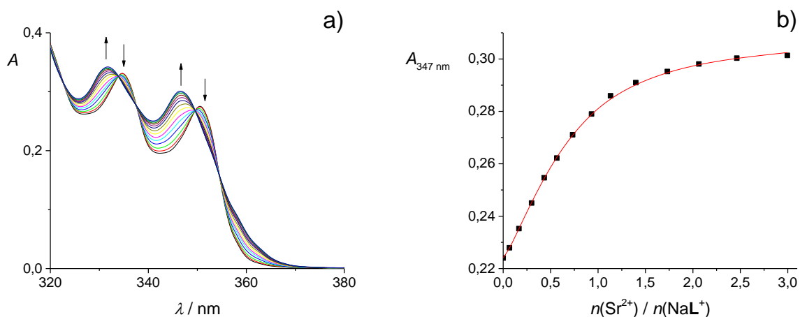
Slika 14. a) Spektrofotometrijska titracija kompleksa \text{NaL}^+ ( c = 9,99 \times 10^{-5} \text{ mol dm}^{-3} ) sa \text{Sr}(\text{ClO}_4)_2 \times 3\text{H}_2\text{O} ( c = 1,46 \times 10^{-3} \text{ mol dm}^{-3} ) u acetonitrilu; \vartheta = (25,0 \pm 0,1) \text{ }^\circ\text{C} ; V(\text{NaL}^+) = 2,2 \text{ cm}^3 ; l = 1 \text{ cm} . Spektri su korigirani za razrjeđenje. b) Ovisnost apsorbancije otopine spoja L pri 347 nm o omjeru množina dodanog \text{Sr}(\text{ClO}_4)_2 \times 3\text{H}_2\text{O} i kompleksa \text{NaL}^+ . ■ eksperimentalne vrijednosti; — izračunane vrijednosti.
