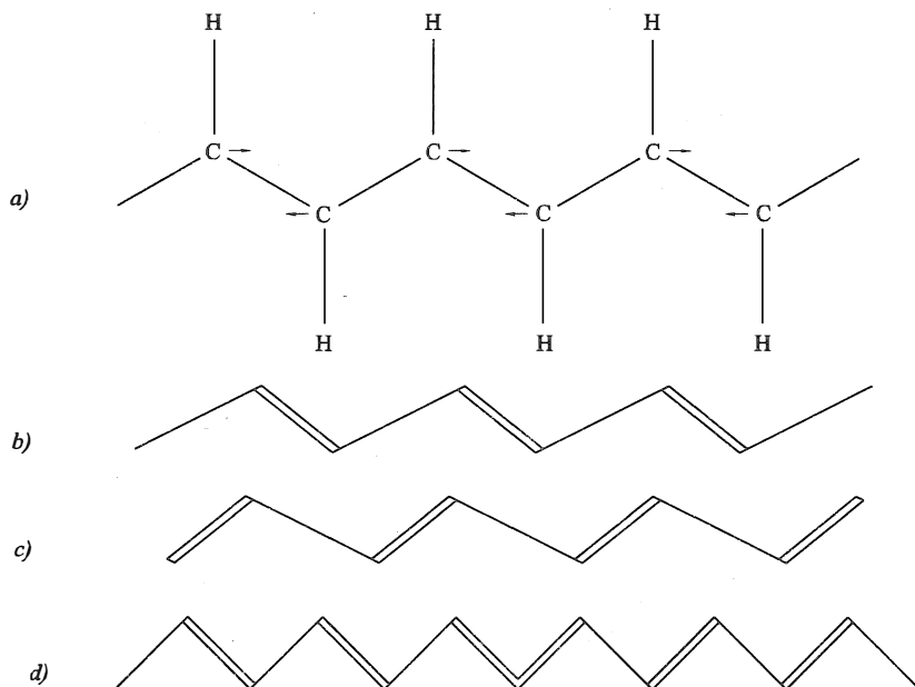
Slika 1. Polimerni lanac (CH)_x , gdje je x broj CH jedinica. Na sl. 1a sve veze među ugljicima su iste. Strjelice pokazuju pomake ugljika kojima se pojavljuje jedna kratka i jedna duga veza sa sl. 1b. Izmjenom predznaka pomaka na sl. 1a nastaje stanje na sl. 1c, jednakopravno je stanje sa sl. 1b. Na sl. 1d stanje 1b ide do pola, a 1c od pola lanca i stvara se prijelazno područje s dvije kratke veze.
