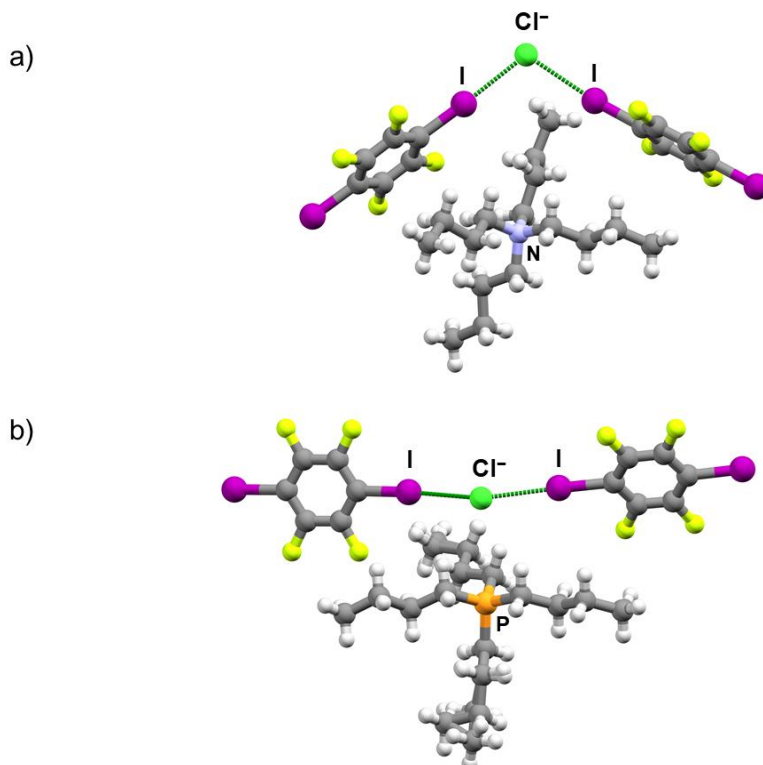
Slika 11. Prikaz povezivanja molekula 14tfib i formulskih jedinica kvaterne amonijeve ili fosfonijeve kloridne soli halogenskom vezom I...Cl - : a) OHOVUD i b) PESRUC (halogenske veze prikazane su zelenom isprekidanom linijom; slika izrađena prema podacima iz ref. 89 i 90)
