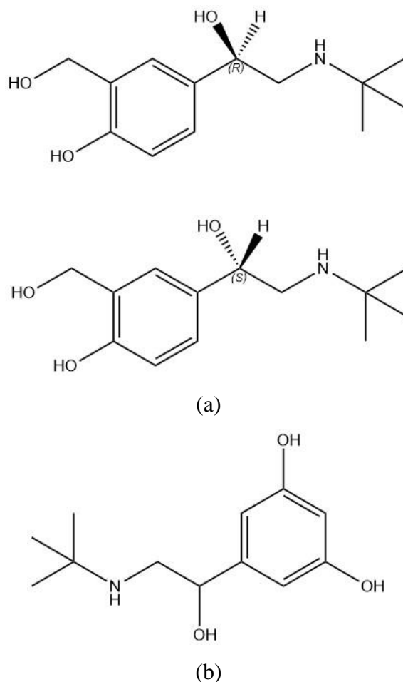
Slika 3. Molekularna struktura beta-2 agonista (a) R - i S -sabutamola i (b)tertbutalina
