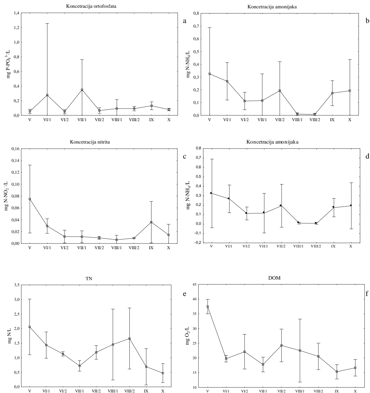
Slika 4 Statistički značajne (Kruskal–Wallis, p < 0,05 ) vremenske promjene analiziranih čimbenika: a) ortofosfata (mg P-PO 4 3- /L), b) koncentracije amonijaka (mg N-NH 4 /L), c) nitrita (mg N-NO 2 - /L), d) nitrata (N-NO 3 - /L), e) TN (mg N/L) i f) DOM (mg O 2 Mn/L) Legenda: \bar{x} \pm SD
