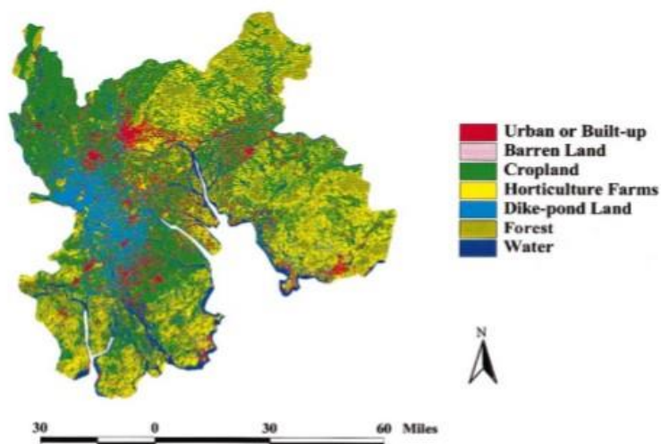
Sl. 8. Korištenje zemljišta i vegetacijski pokrov u delti rijeke Zhujiang, 1989. godine Izvor: Land use change analysis in the Zhujiang Delta of China using satellite remote sensing, GIS and stochastic modelling
