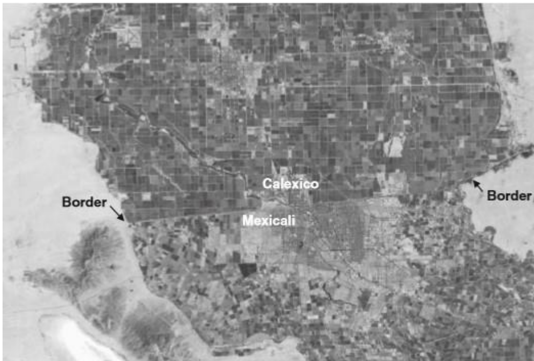
Sl. 11. Kompozitna slika Landsat ETM + u boji nastala 3. svibnja 2000. u pograničnom području
