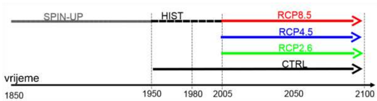
Slika 6. Shematski prikaz trajanja pojedinih simulacija spregnutog atmosfersko-oceanskog modela buduće klime CNRM-RCSM4.
