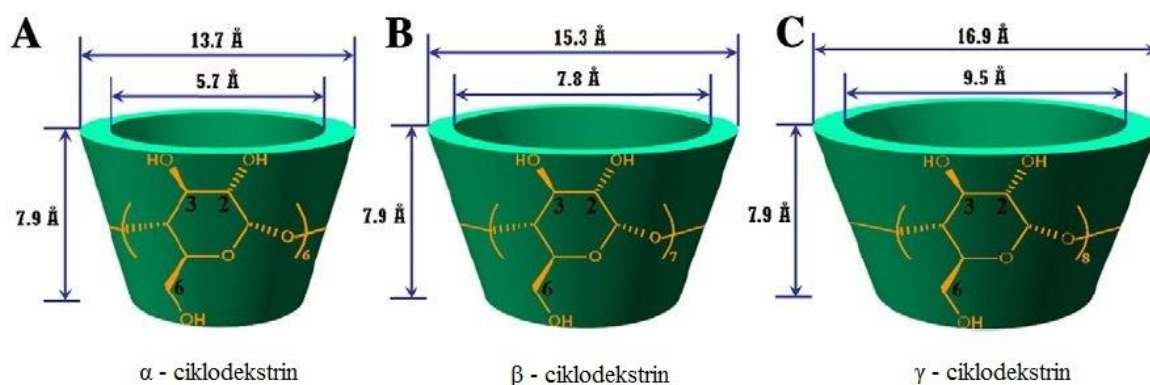
Slika 5. Struktura i dimenzije prirodnih ciklodekstrina ( \alpha , \beta i \gamma ciklodekstrini). 66
