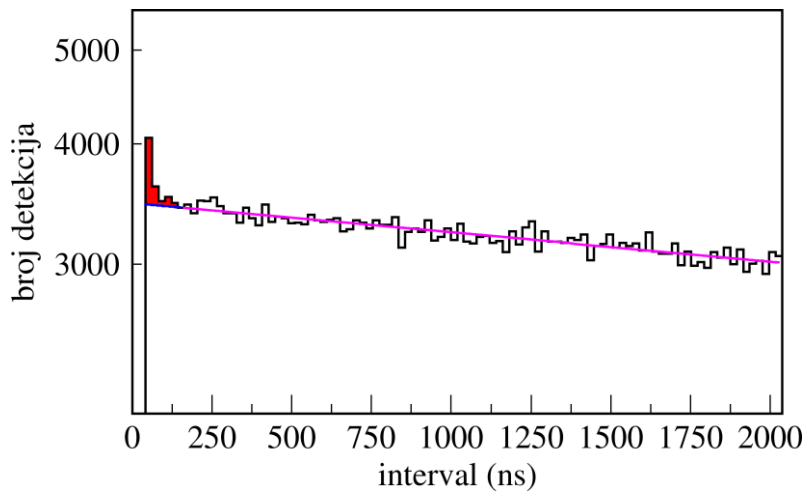
Slika 5.3. Distribucija vremena čekanja za tamne događaje fotodiode I5293 pri 10 V prekonaponu, prije zračenja. Ljubičasti pravac predstavlja fit eksponencijalne krivulje na tamne događaje a plava dužina je njegovo produljenje u područje gdje očekujemo afterpulseve. Crveno područje popularaju afterpulsevi. Prema izračunu (vidi tekst) vjerojatnost afterpulsu je (0.00041 \pm 0.00001) odnosno 0.041%.
