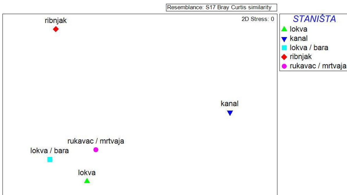
Slika 35. Prikaz rezultata multivarijantne analize (NMDS) ( \log(x+1) transformirani podaci) uz superponirane rezultate klaster analize temeljene na Bray-Curtisovom koeficijentu sličnosti ( group average linking ) u sastavu zajednica vodenih kornjaša istraživanih staništa.
