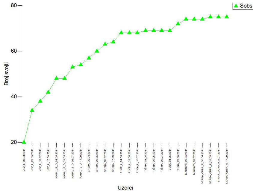
Slika 25. Akumulacijska krivulja povećanja kumulativnog broja svojti vodenih kornjaša na istraživanim lokalitetima.
