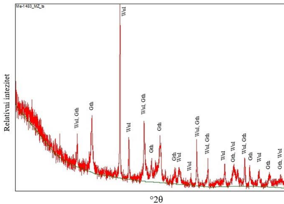
Slika 35. Difraktogram uzorka Me1483 MZ-ts s naznačenim fazama koje su prisutne u uzorku.
