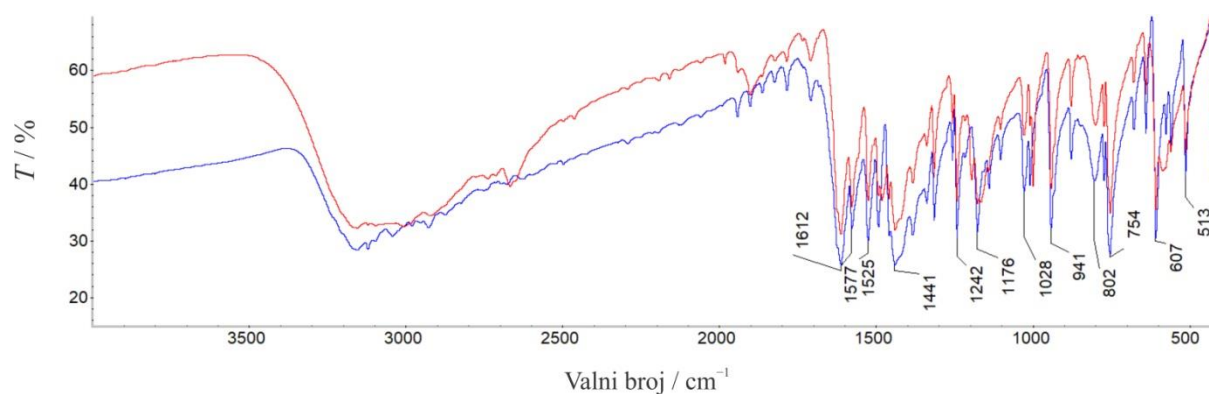
Slika 30. FTIR spektri reakcijske smjese spoja H (plavi spektar), te spoja H , hidroksilamonijevog klorida i katalitičke količine etanola (crveni spektar) nakon 110 minuta mljevenja.
