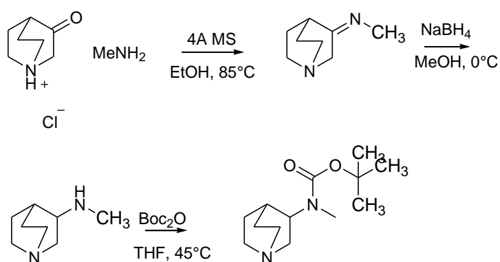
Shema 8. Sintaza amina redukcijom Schiffove baze.
