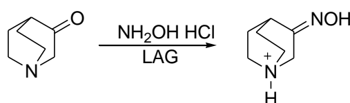
Shema 34. Reakcija pripreve oksima kinuklidin-3-ona mehanokemijski bez dodatka baze
