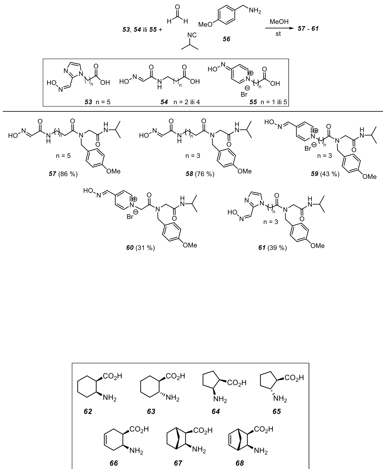
Slika 8. Bifunkcionalni spojevi za pripremu \beta -laktamskih derivata 69 – 77 Ugijevom reakcijom.
