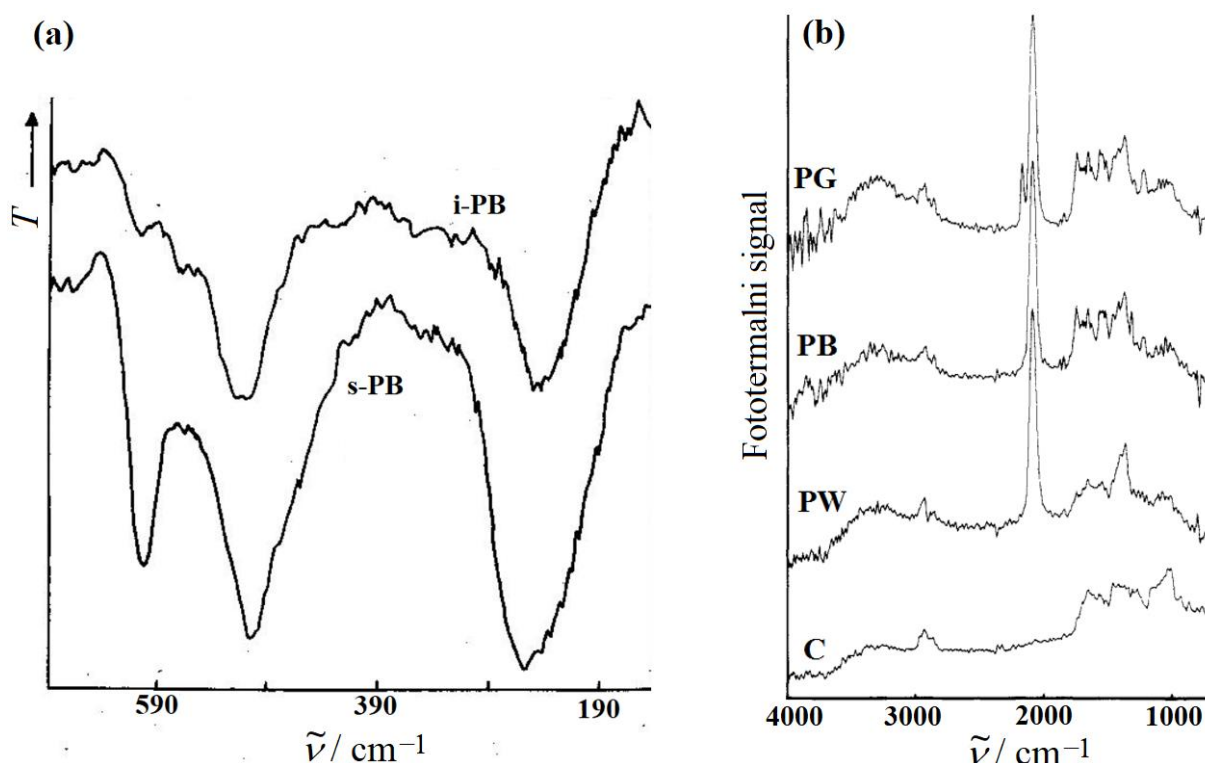
Slika 2.5. (a) Spektri kemijski sintetiziranog topljivog (s-PB) i netopljivog (i-PB) berlinskog modrila u dalekom infracrvenom području; (b) FTIR spektri filмова topljivog berlinskog modrila (PB) te njegove reducirane (PW) i oksidirane (PG) forme. Oznakon C obilježen je FTIR spektar grafitne elektrode.
