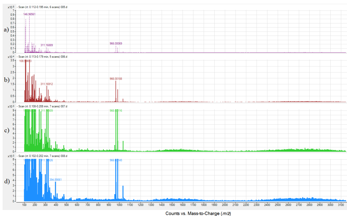
Slika D14 . Spektri masa otopina pripravljenih otapanjem prethodno izoliranih kompleksa: PZQ- \beta -CD (a), PZQ-HP- \beta -CD (b), PZQ-SBE- \beta -CD (c) i PZQ-RM- \beta -CD (d) snimljeni u negativnom načinu rada.
