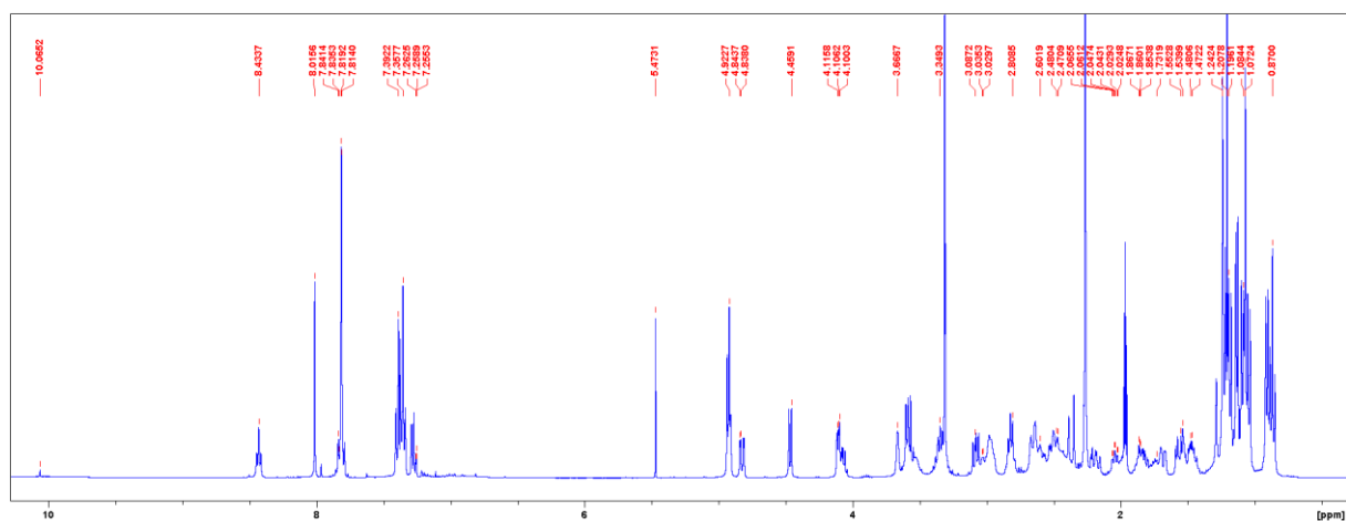
D4. Spektar 1 H NMR spoja f1 .
